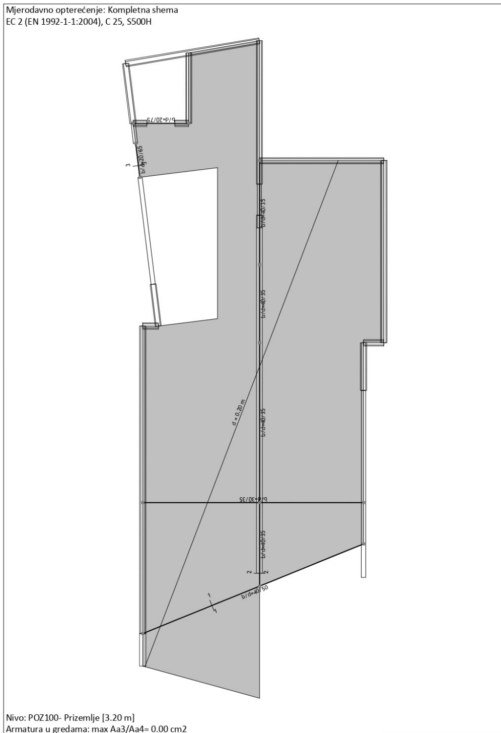
Slika 92. Potrebna armatura za grede POZ100
