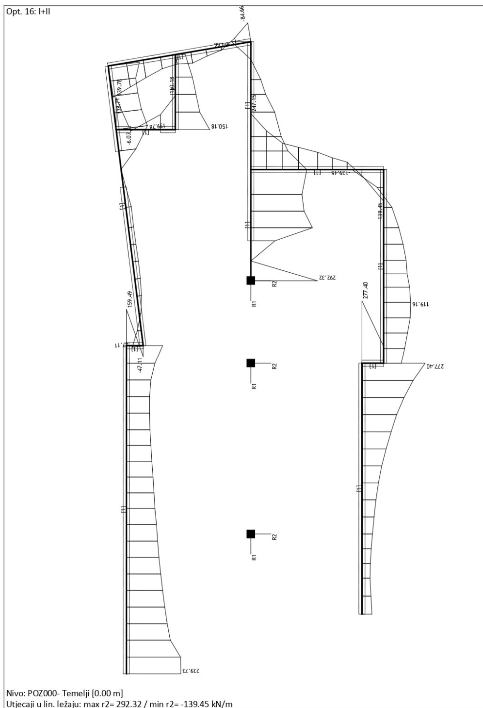
Slika 75. Linijske reakcije u ležajevima POZ000 za GSN
