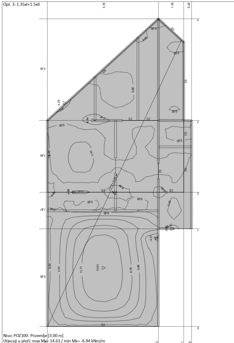
Slika 118. Momenti savijanja M_x u ploči POZ100 – GSN
