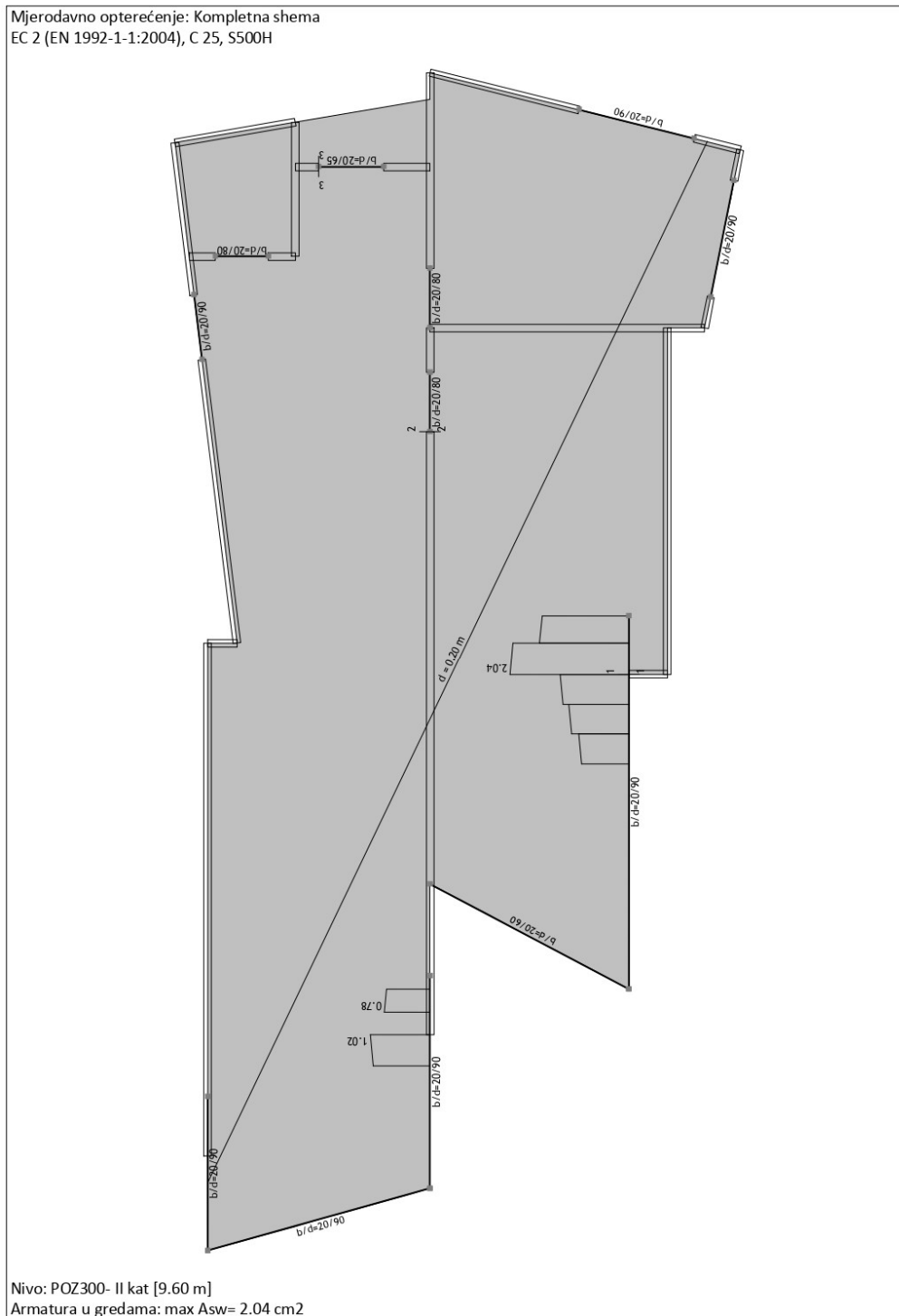
Slika 87. Potrebna poprečna armatura za grede POZ300
