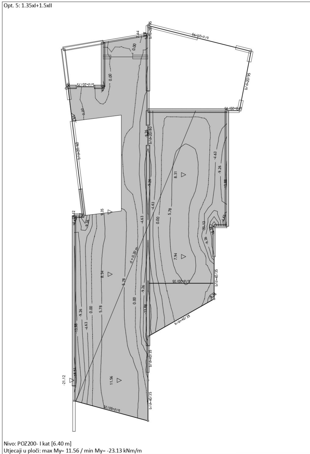
Slika 47. Momenti savijanja M_y u ploči POZ200 – GSN
