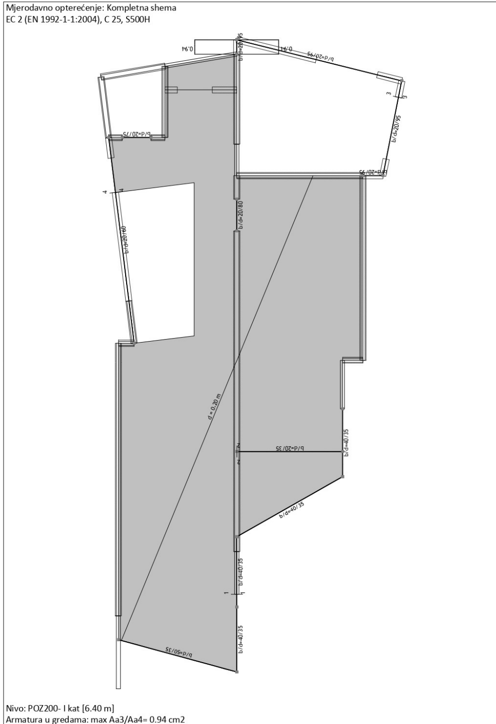
Slika 89. Potrebna armatura za grede POZ200
