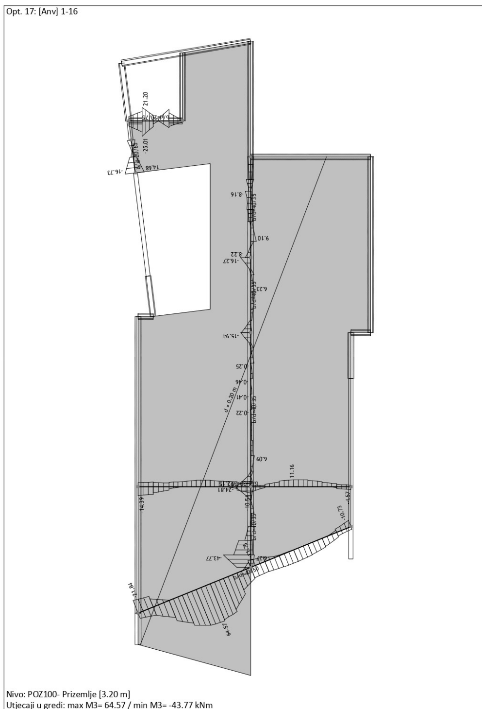
Slika 56. Momenti savijanja M za grede POZ100 – GSN
