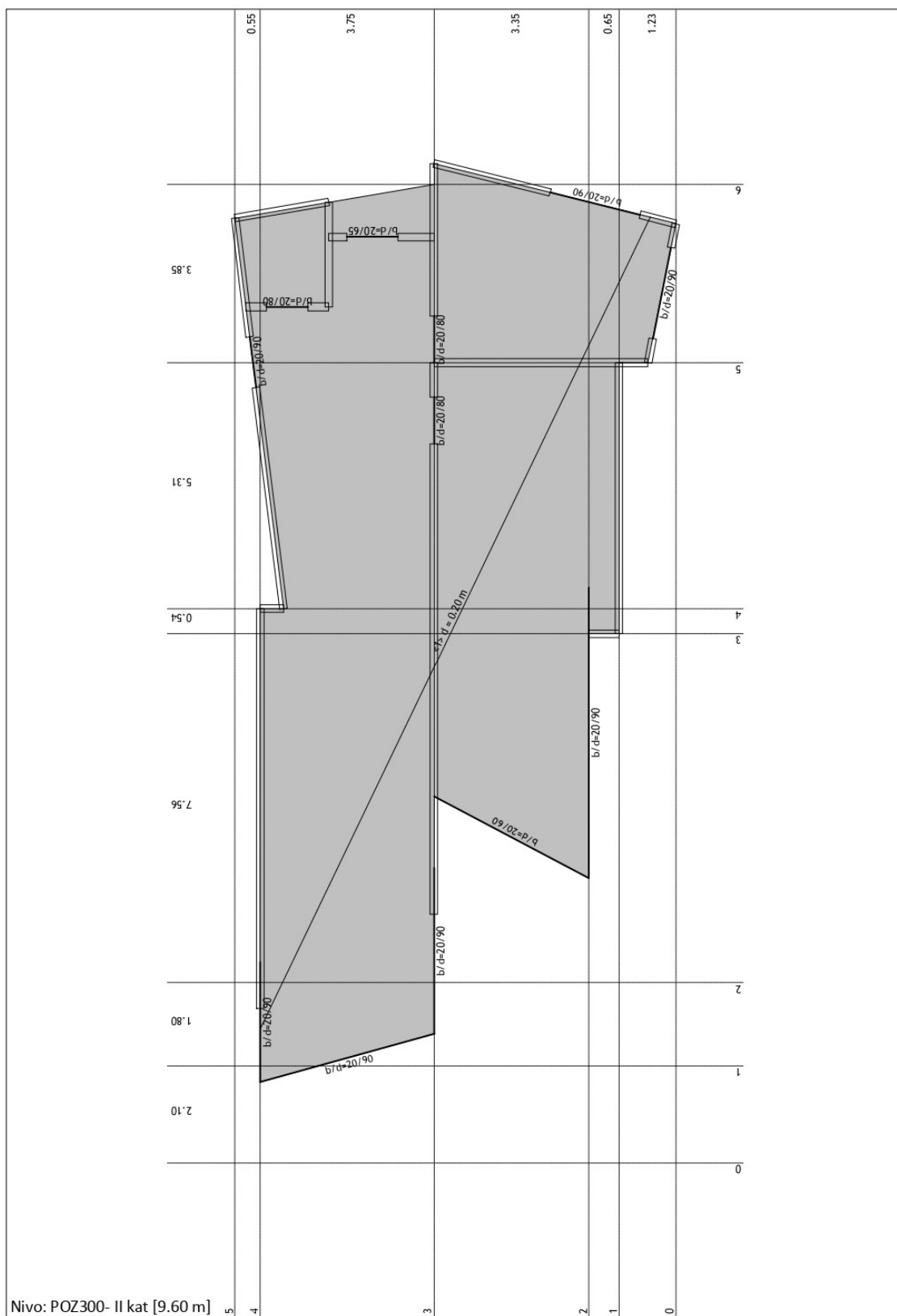
Slika 11. Plan pozicija 300
