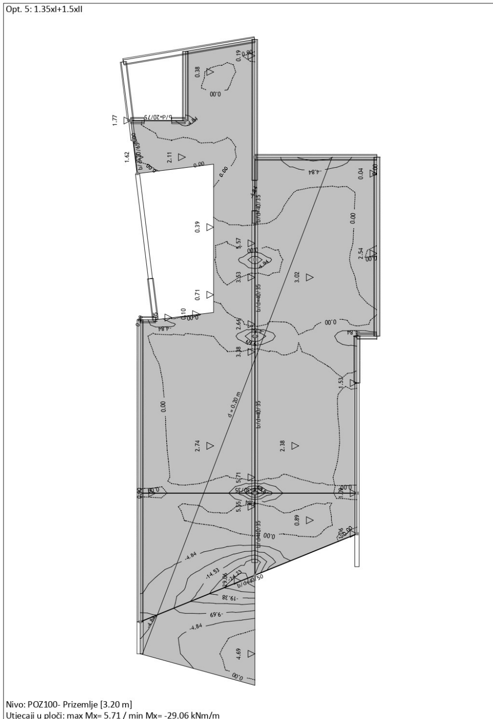
Slika 53. Momenti savijanja M_x u ploči POZ100 – GSN
