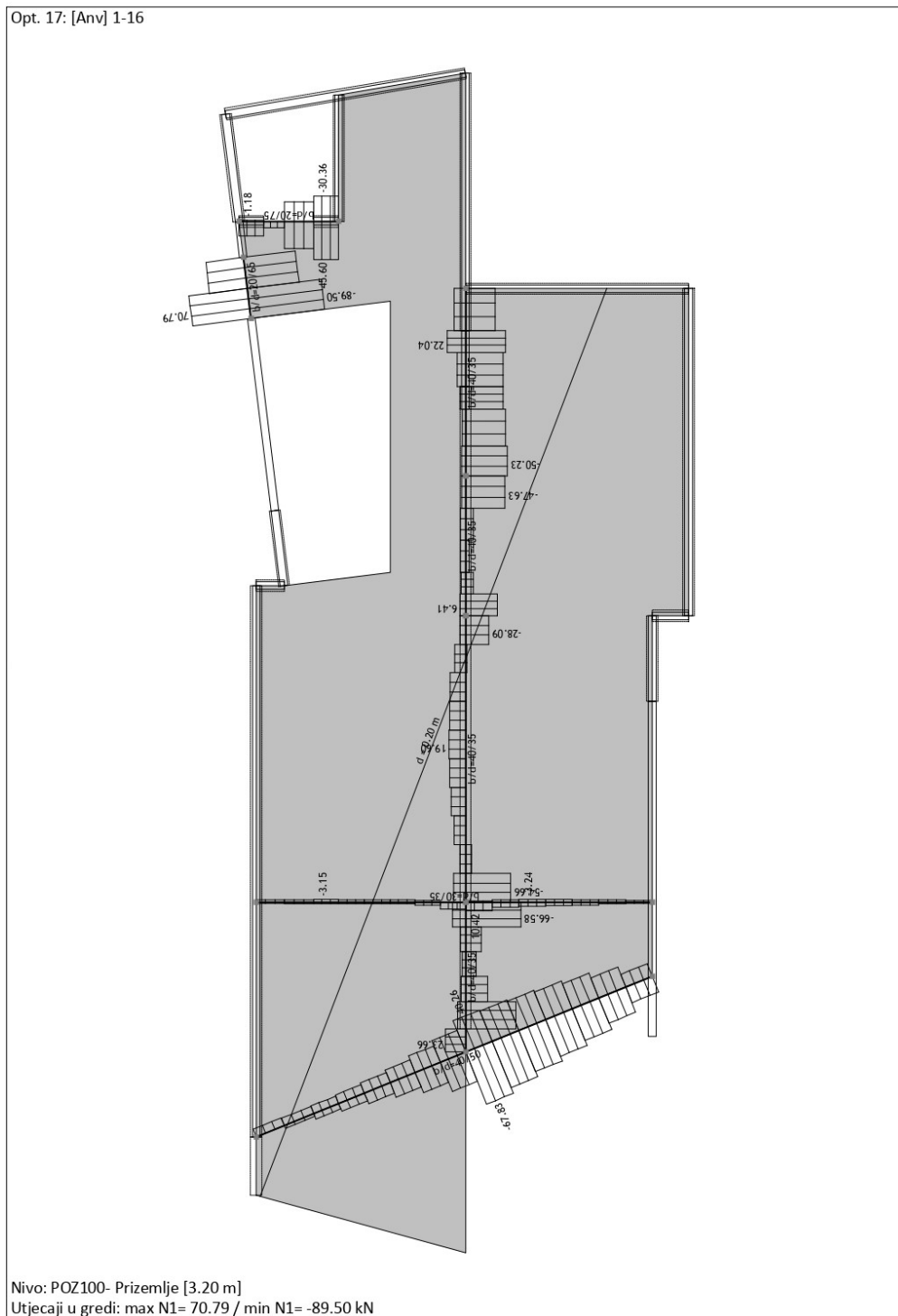
Slika 58. Uzdužne sile N za grede POZ100 – GSN
