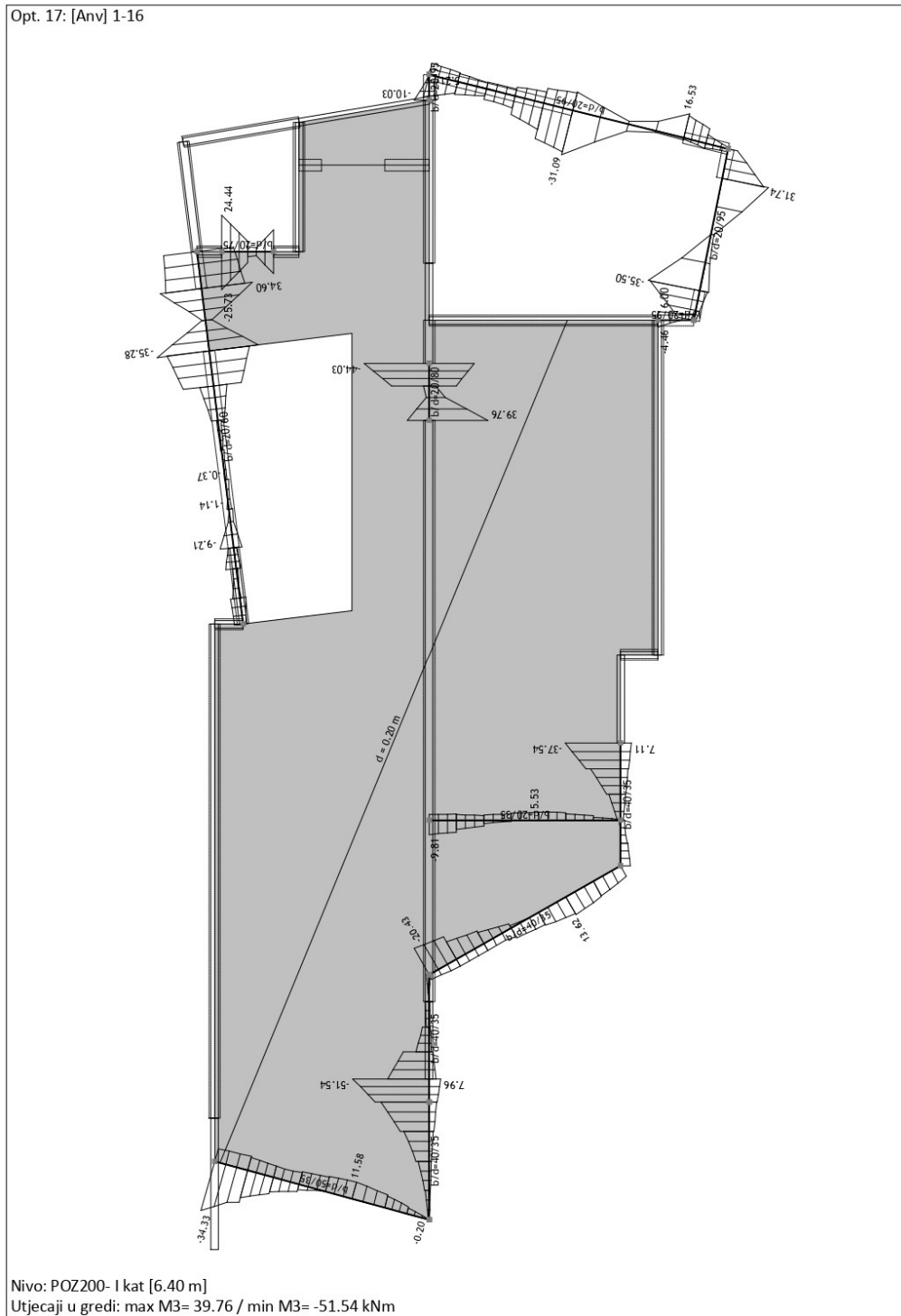
Slika 49. Momenti savijanja M za grede POZ200 – GSN
