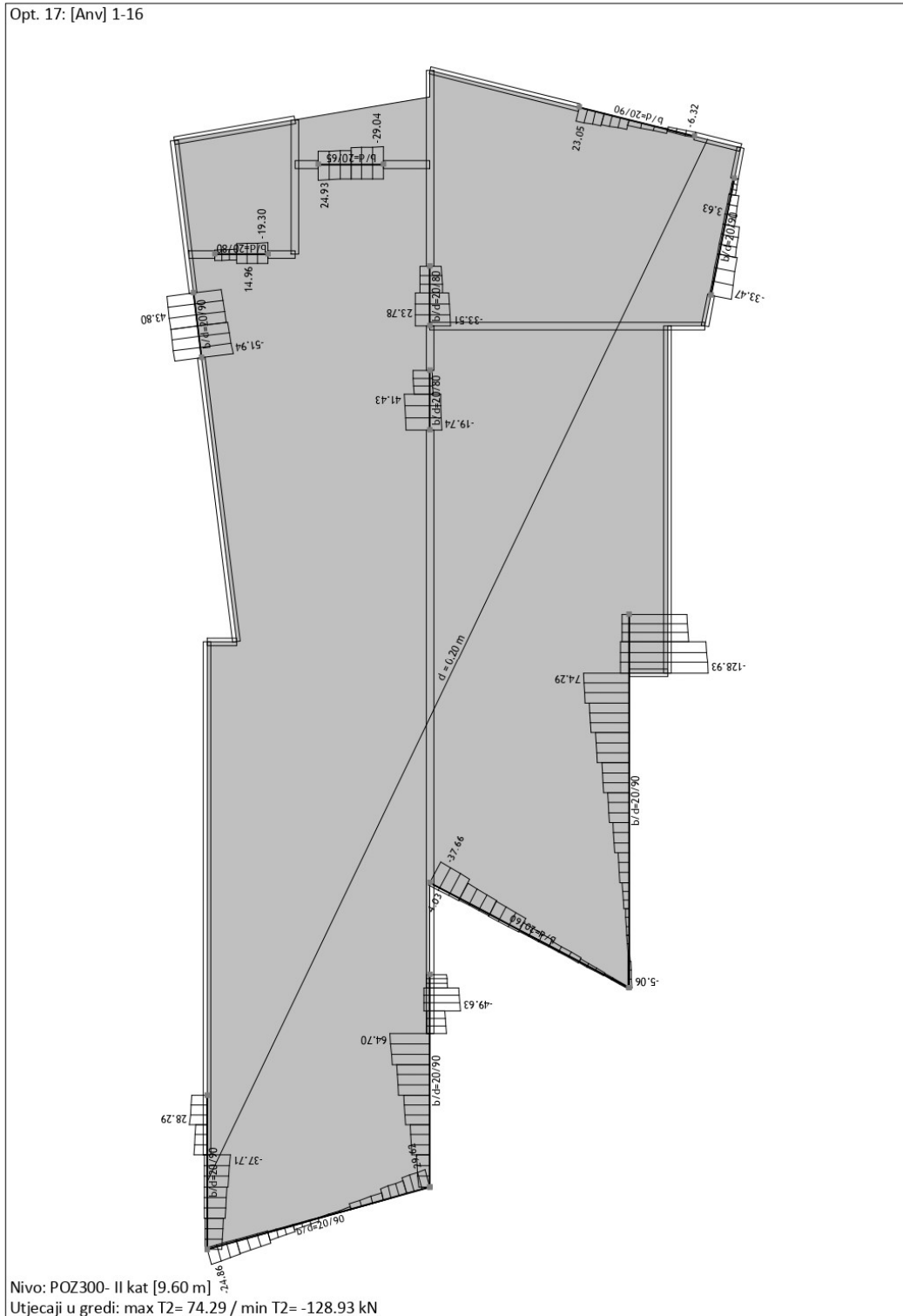
Slika 43. Poprečne sile T za grede POZ300 – GSN
