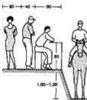
13 Prikladan ophod za gledatelje
