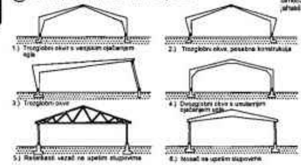
3 Poprečni presjeci hala
