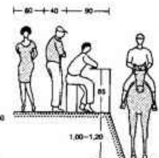
12 Profil ograde
