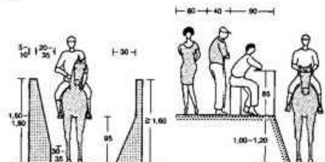
12 Profil ograde
