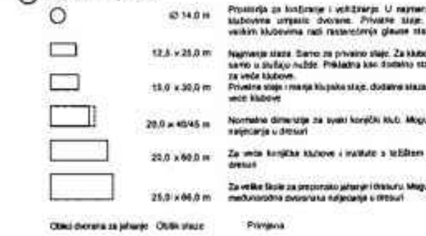
4 Svjetle mjere dvorane za jahanje
