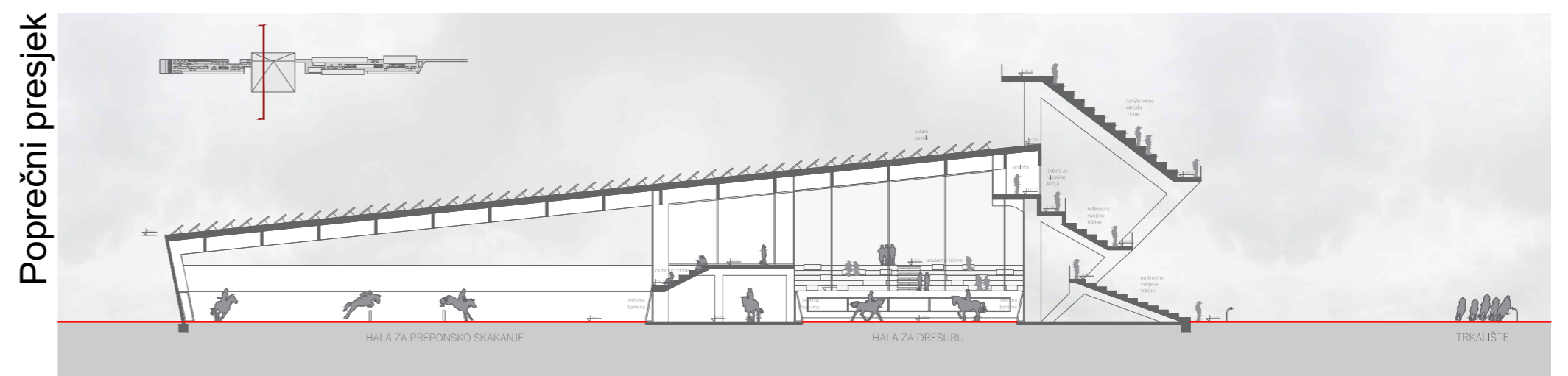
Dijagramski presjeci
