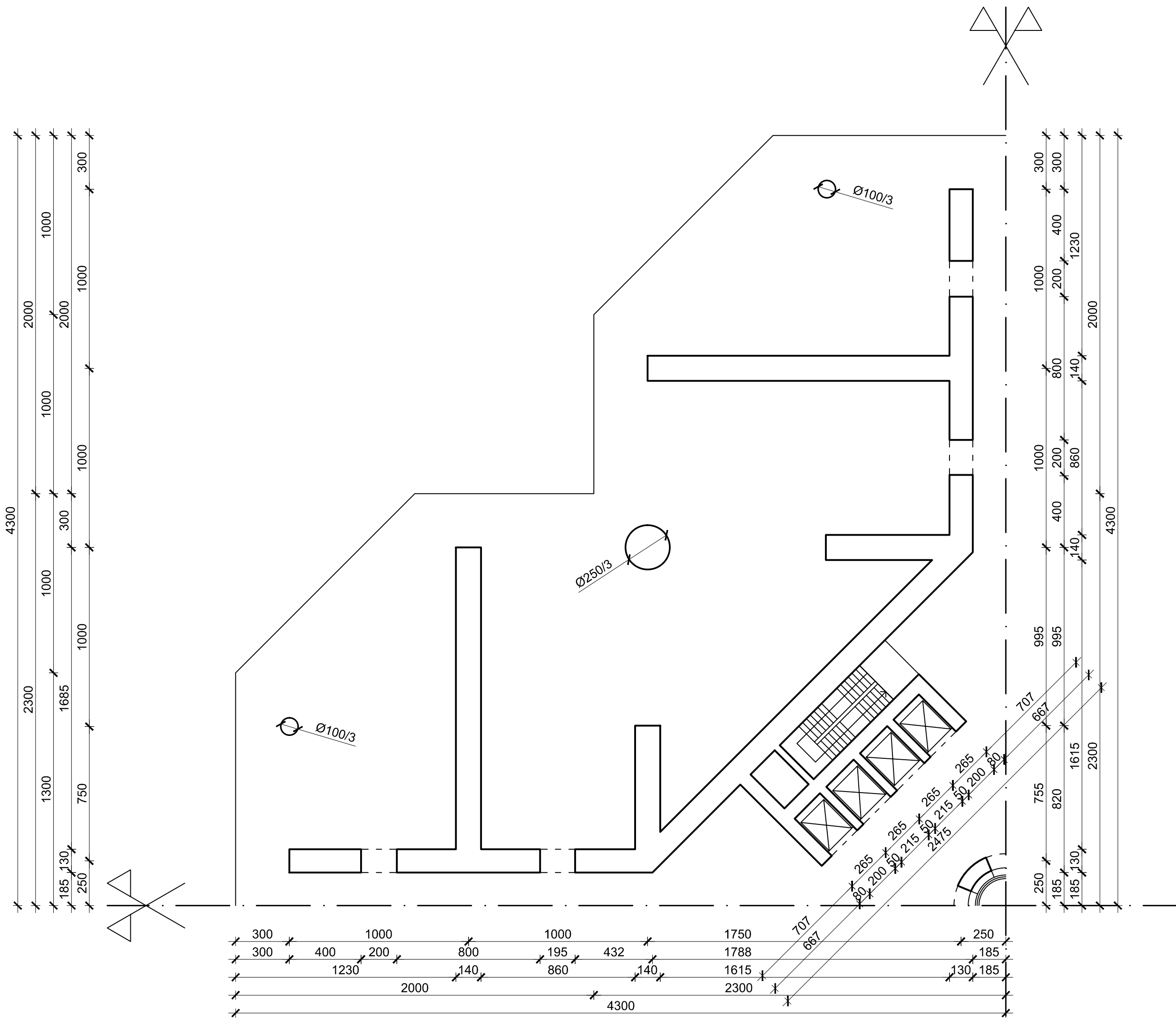
TLOCRT SEGMENTA - RAZINA 300-500 m M 1:200
