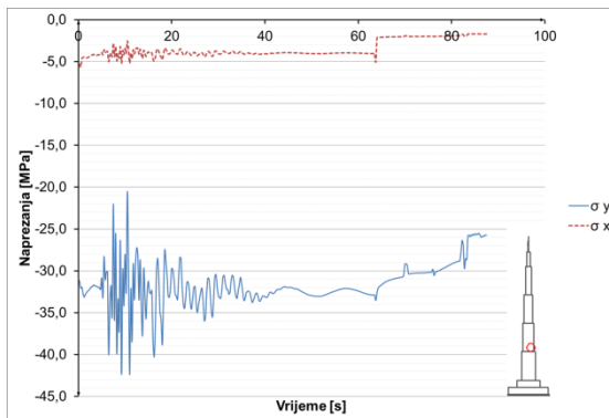
Slika 8.3.4.21 Naprezanja u betonu u presjeku h=305 m – potres Kobe
