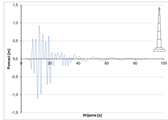
Slika 8.3.4.15 Pomaci u presjeku h=1052 m – potres Kobe
