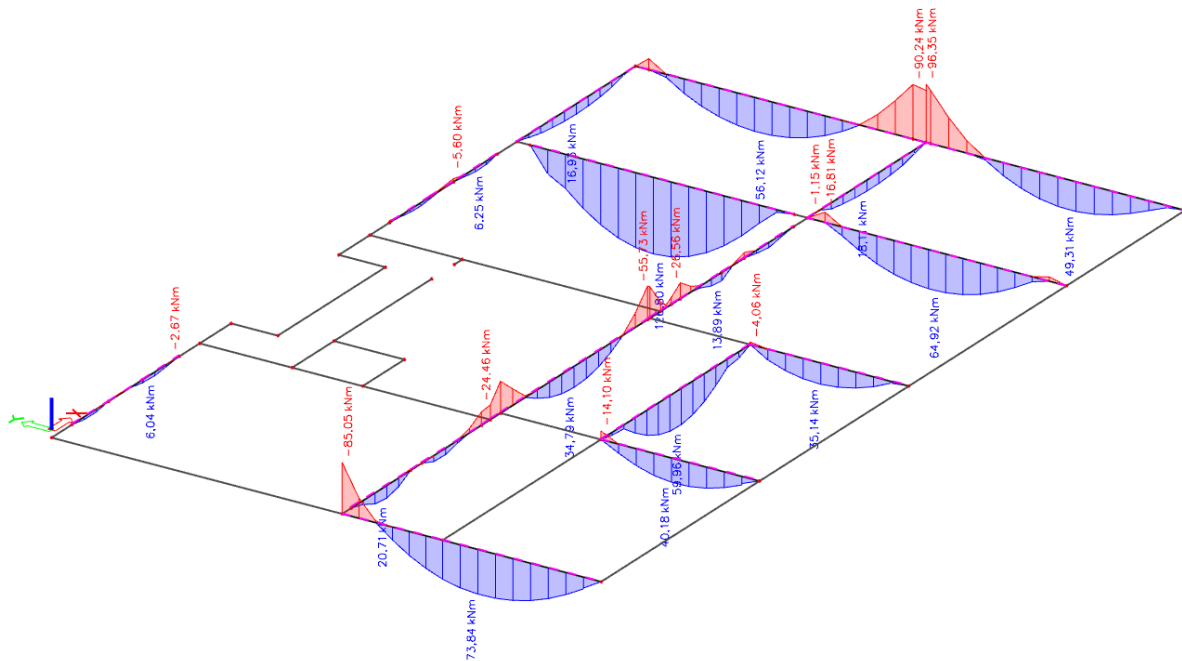
Slika 5.72. Momenti savijanja M_{Ed,y} [kNm] za GSU_2
