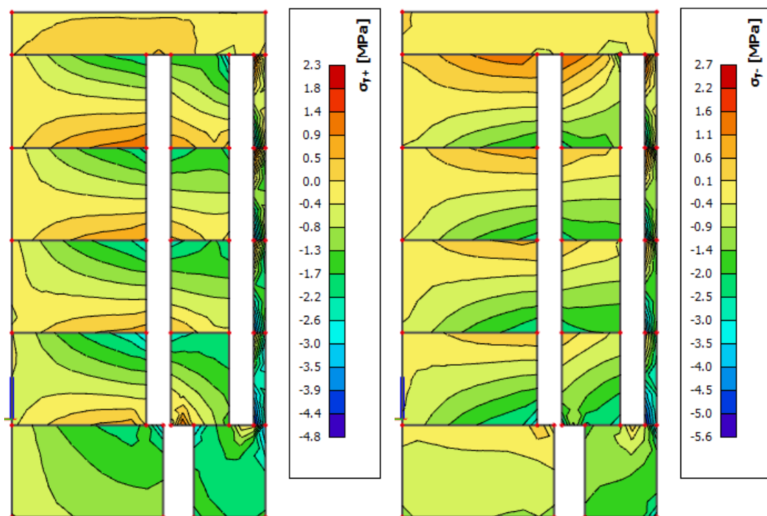
Slika 6.9. Napreznja u y smjeru (za zidove od betona C25/30; \sigma_{c,Ed} \leq 0,45 \cdot f_{ck} = 11,25 \text{ MPa} )
