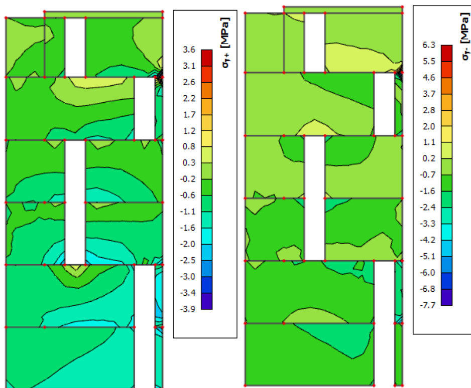
Slika 6.54. Napreznja u y smjeru (za zidove od betona C25/30; \sigma_{c,Ed} \leq 0,45 \cdot f_{ck} = 11,25 \text{ MPa} )
