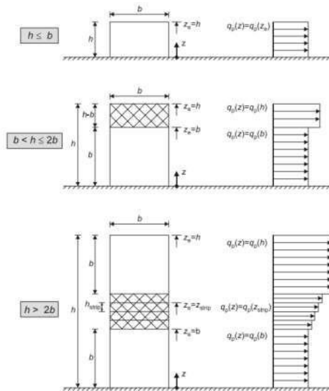
Slika 2.4. Referentna visina z_e u ovisnosti h/b te odgovarajući profil pritiska
