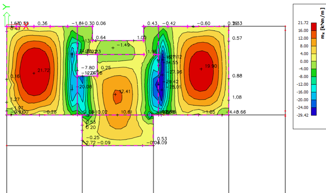
Slika 5.68. Momenti savijanja M_{Ed,x} [kNm/m] za GSU ( 1.0 \cdot G + 1.0 \cdot Q )
