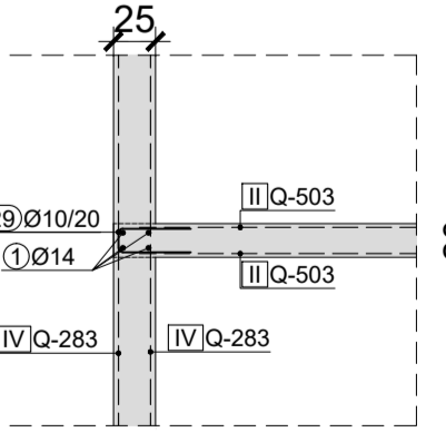
spoj ploče i zida
