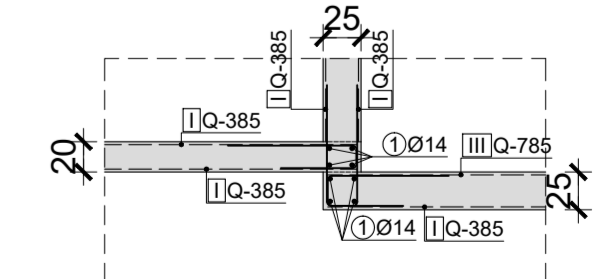
PRESJEK 1-1
