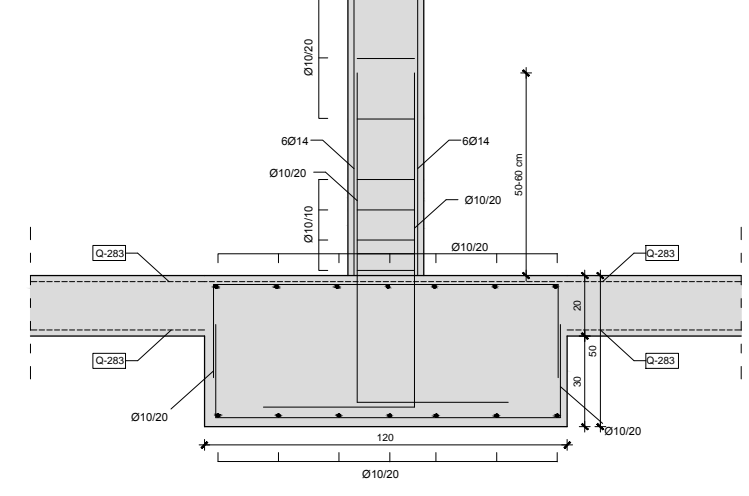
PRESJEK C-C M 1:25
