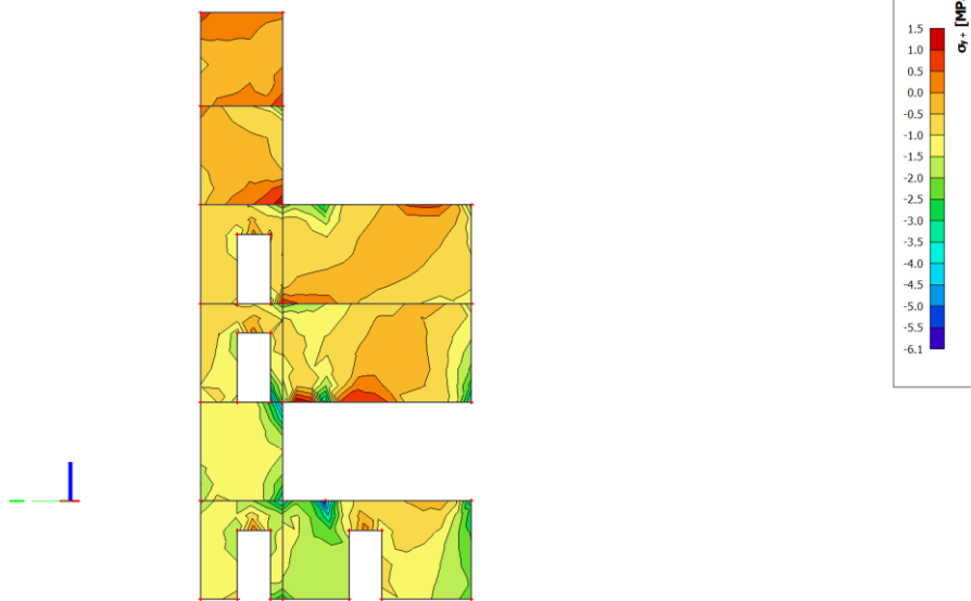
Slika 9.1.37. Naprezanja \sigma_y za anvelopu opterećenja (GSNSX+GSNSY+GSN)
