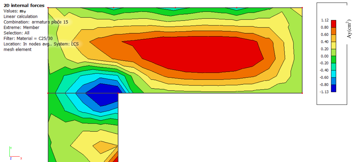
Slika 8.1.38. Armatura ploče d=15 cm smjer y-y za GSN
