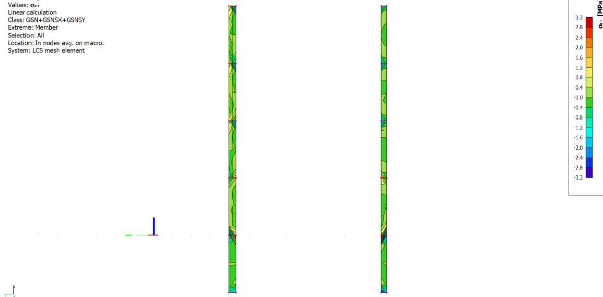
Slika 9.1.16. Naprezanja \sigma_x za anvelopu opterećenja (GSNSX+GSNSY+GSN)
