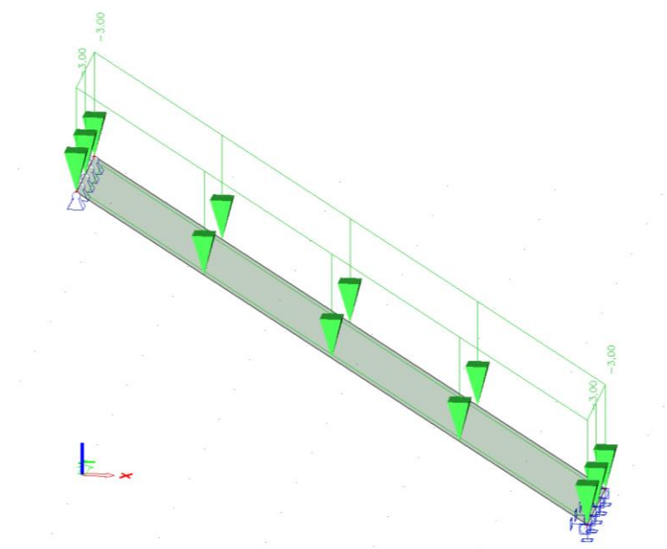
Slika 6.14. Promjenjivo opterećenje
