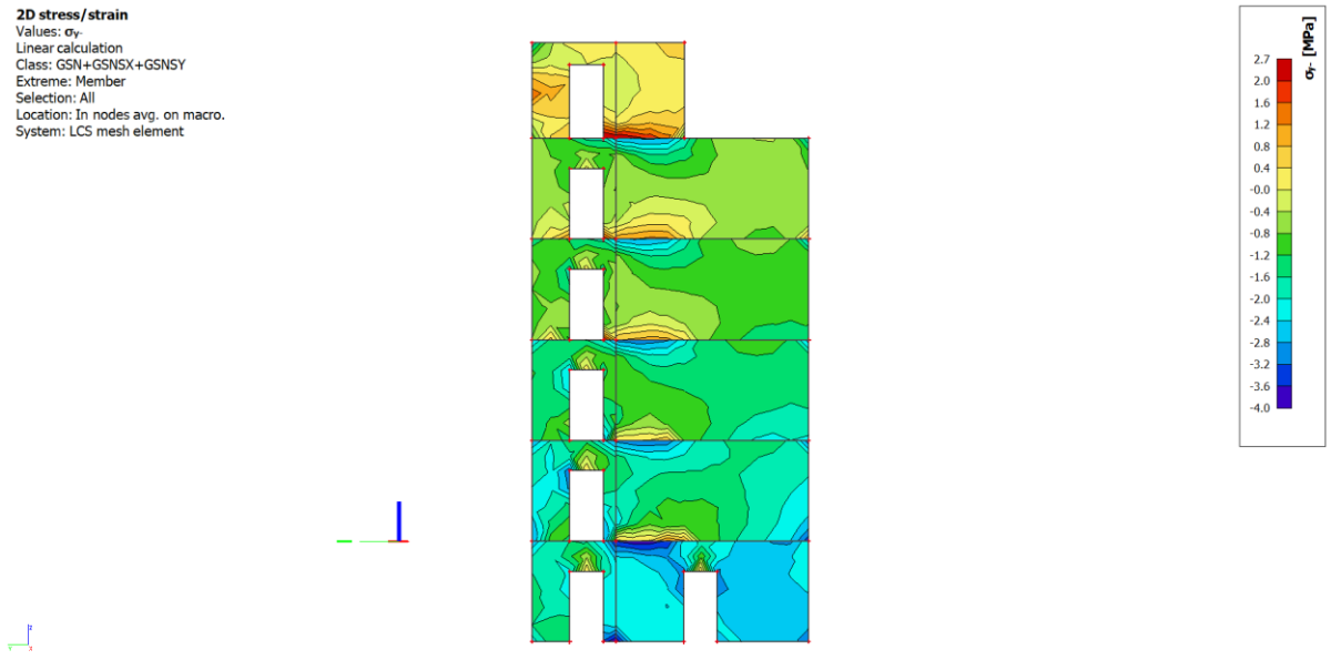
Slika 9.1.22. Naprezanja \sigma_y za anvelopu opterećenja (GSNSX+GSNSY+GSN)
