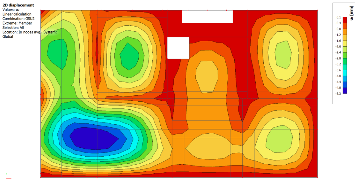
Slika 8.1.2. Progibi ploča [mm] za GSU-2 ( \delta EL \leq L/1250 )
