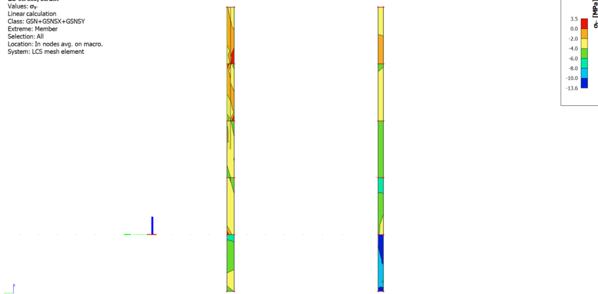
Slika 9.1.17. Naprezanja \sigma_y za anvelopu opterećenja (GSNSX+GSNSY+GSN)
