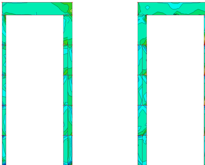
Slika 9.1.13. Naprezanja \sigma_1 za anvelopu opterećenja (GSNSX+GSNSY+GSN)
