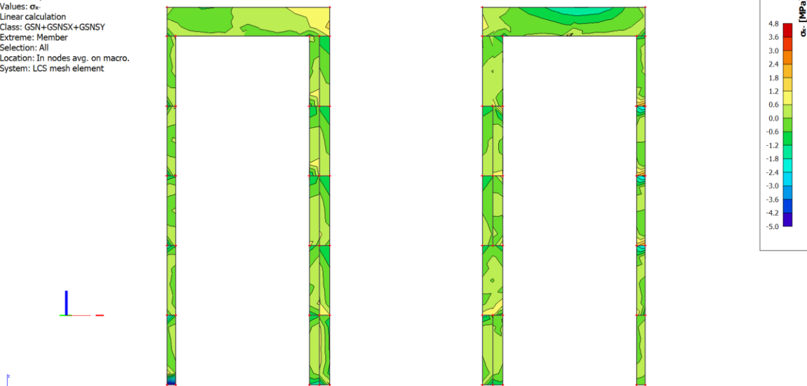
Slika 9.1.11. Naprezanja \sigma_x za anvelopu opterećenja (GSNSX+GSNSY+GSN)
