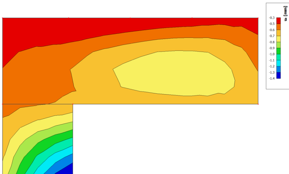
Slika 8.1.34. Progibi ploča [mm] za GSU-2 ( \delta EL \leq L/1250 )
