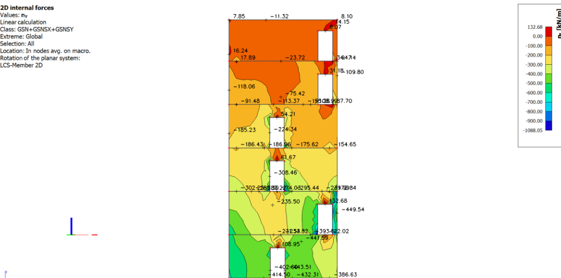
Slika 9.1.10. Uzdužna sila n_x za anvelopu opterećenja (GSNSX+GSNSY+GSN)
