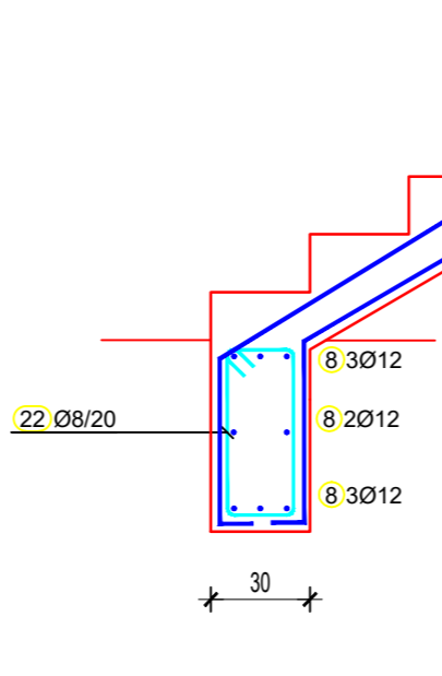
Presjek 3-3 R=1:25
