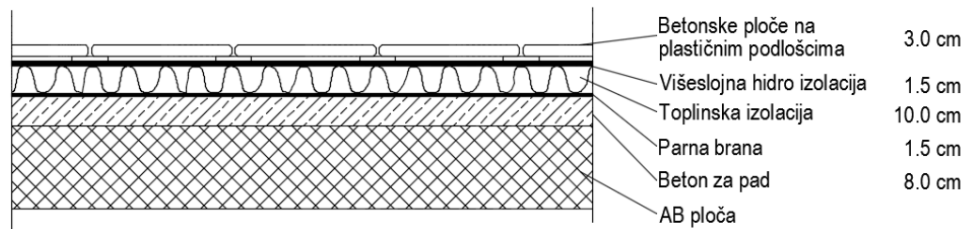
Slika 6.1. Slojevi poda
