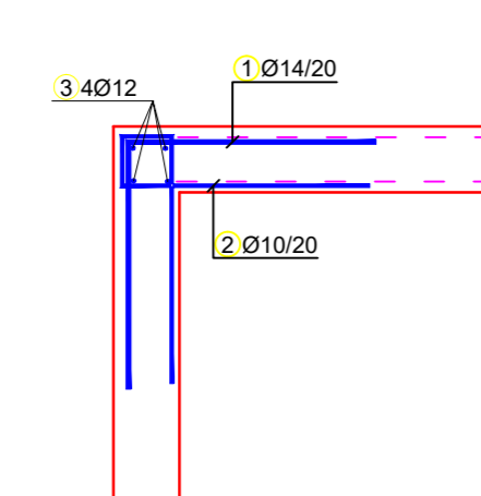
Presjek 1-1 R=1:25
