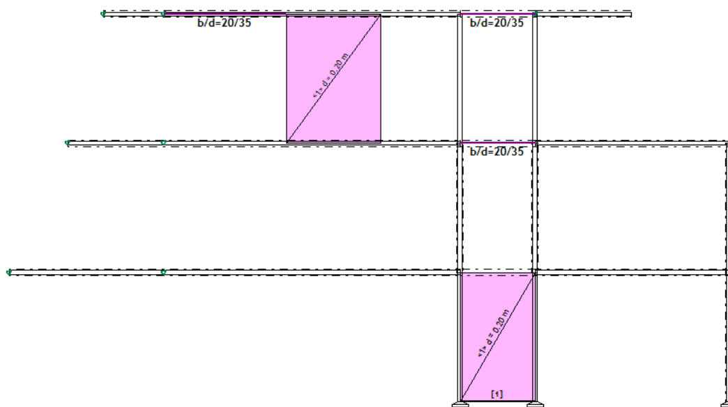
Slika 7.10. Okvir H 6
