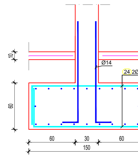
Presjek 2-2 R=1:25
