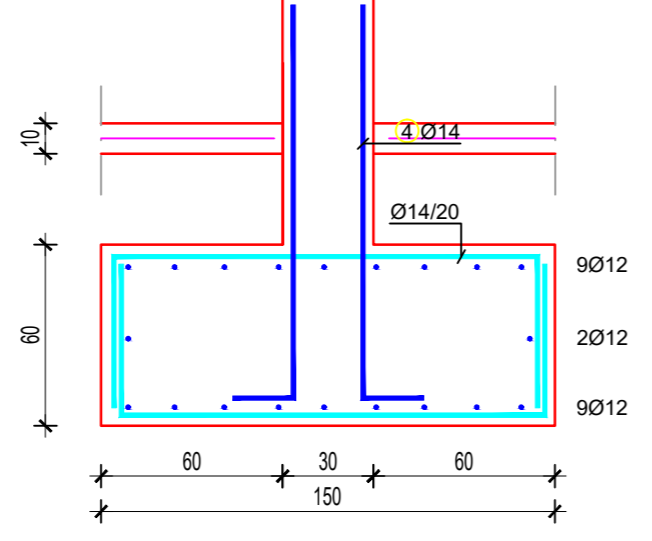
Presjek 2-2 R=1:25
