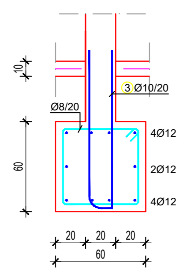
Presjek 1-1 R=1:25
