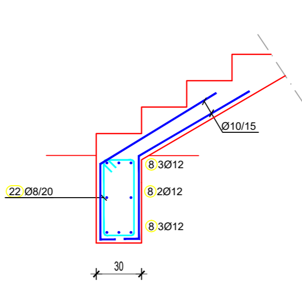
Presjek 3-3 R=1:25
