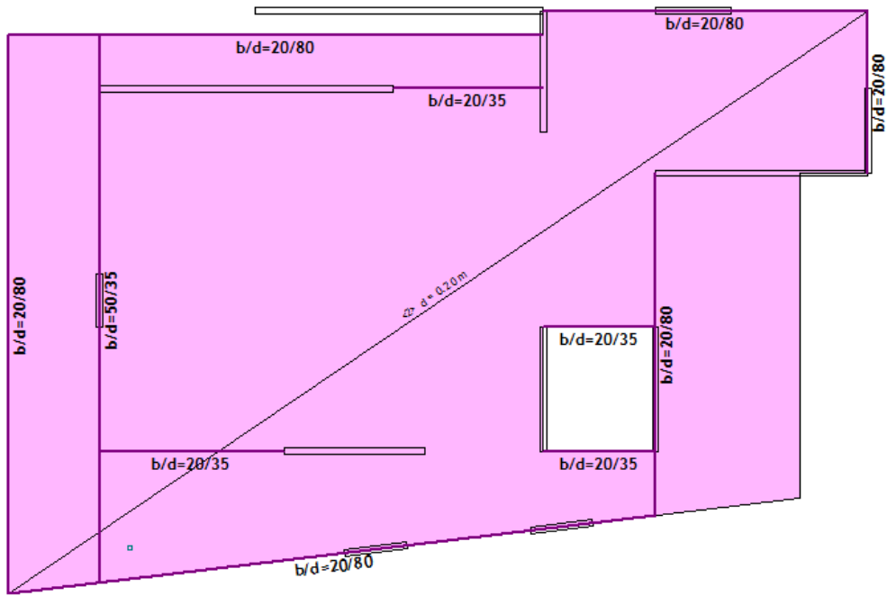
Slika 7.6. Plan pozicije 300
