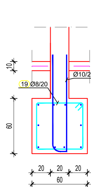
Presjek 1-1 R=1:25
