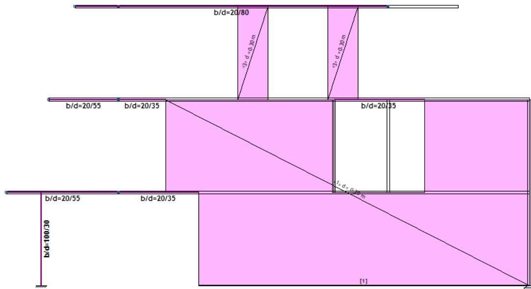
Slika 7.8. Okvir K_1
