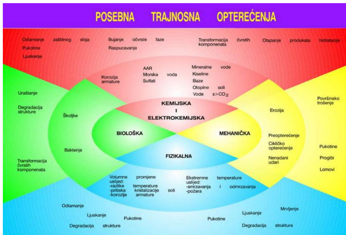
Slika 2.4. Trajnosna opterećenja [10]
