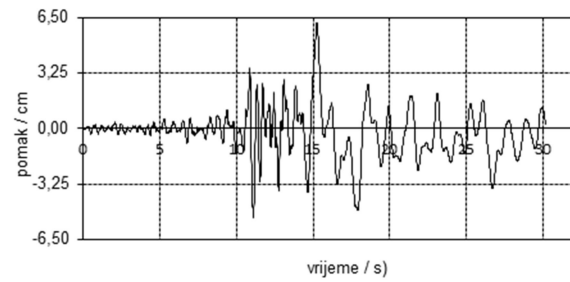
(o) Campano Lucano – vršno ubrzanje a=3.00 g
