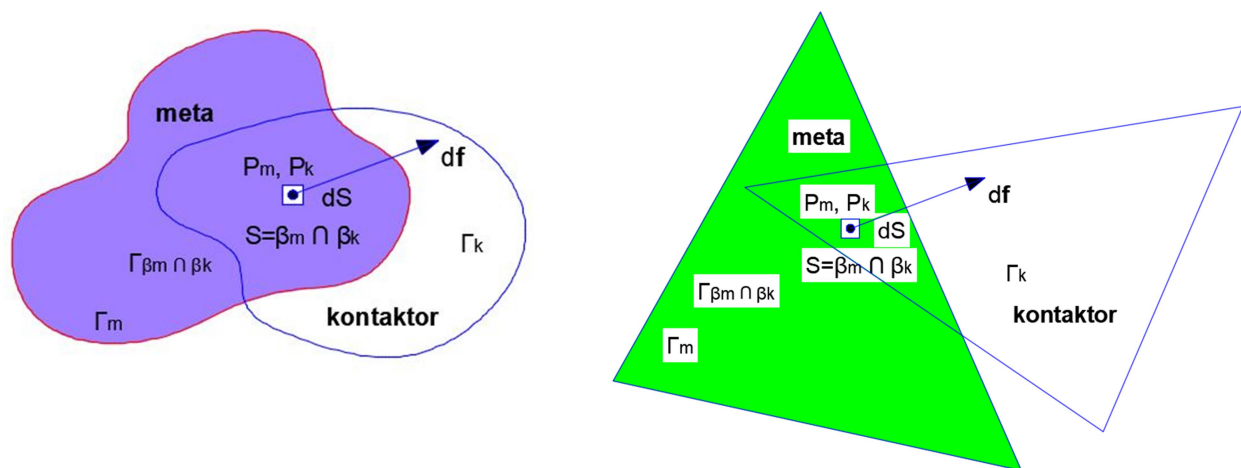
Slika 3. Kontaktna diferencijalna sila u okolini točaka P_m i P_k [6]
