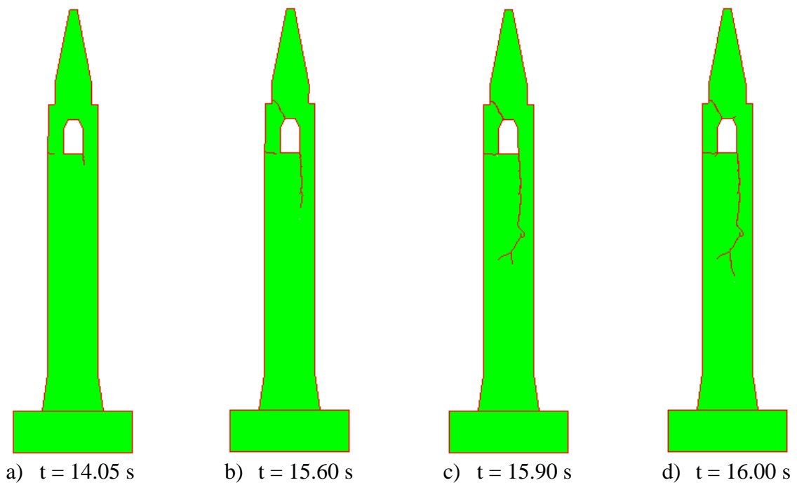
Slika 8. Zvonik izložen djelovanju potresa za ubrzanje 2.00 \text{ g}
