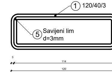
PRESJEK X-X
