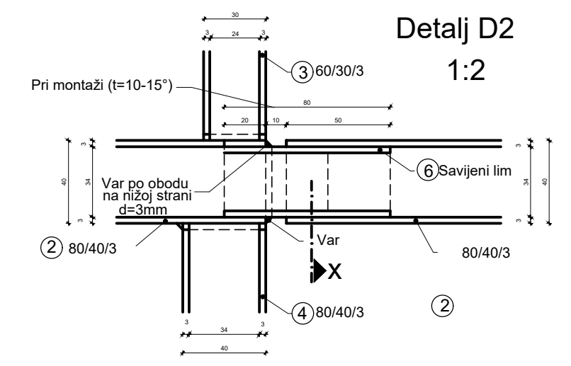
Detalj D 2 1:2
