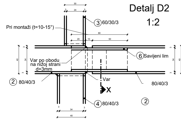
Detalj D 2 1:2
