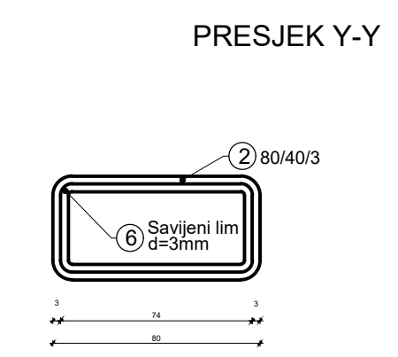
Detalj D2 1:2
