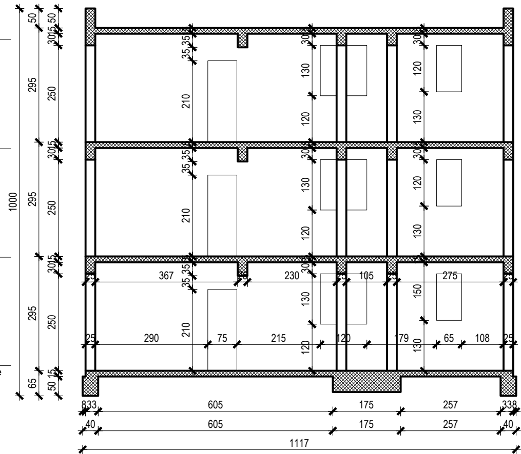
PRESJEK 2-2 M 1:100
