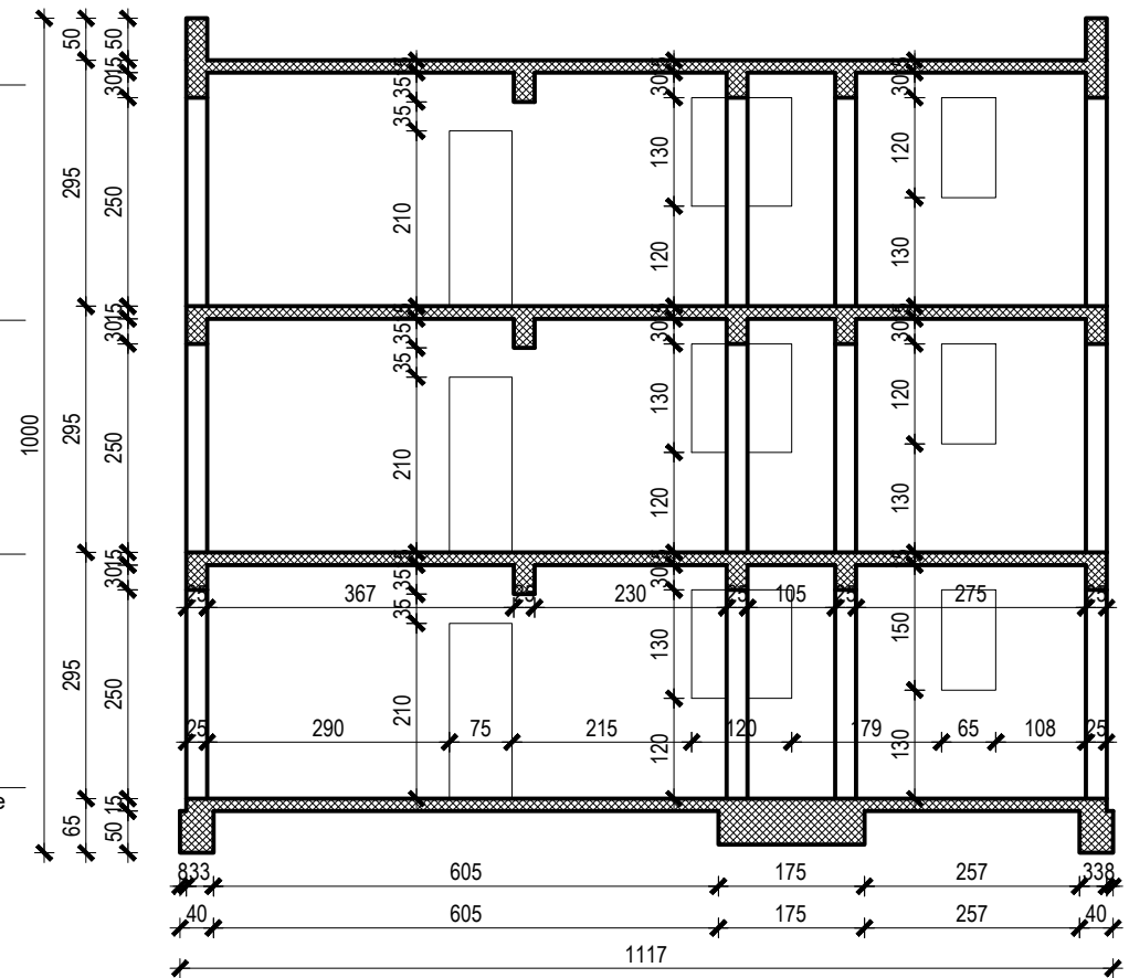
PRESJEK 2-2 M 1:100
