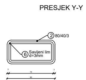
Detalj D2 1:2
