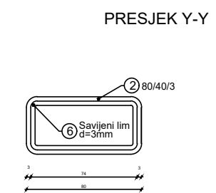
Detalj D2 1:2
