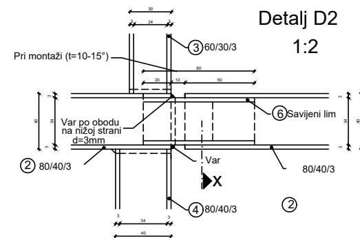
Detalj D 2 1:2
