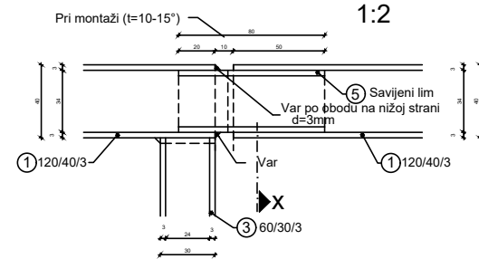
Detalj D 1 1:2
