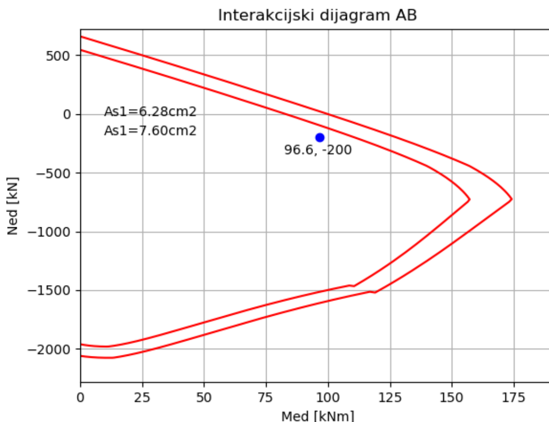
Slika 41: Interakcijski dijagram karakterističnog serklaža
