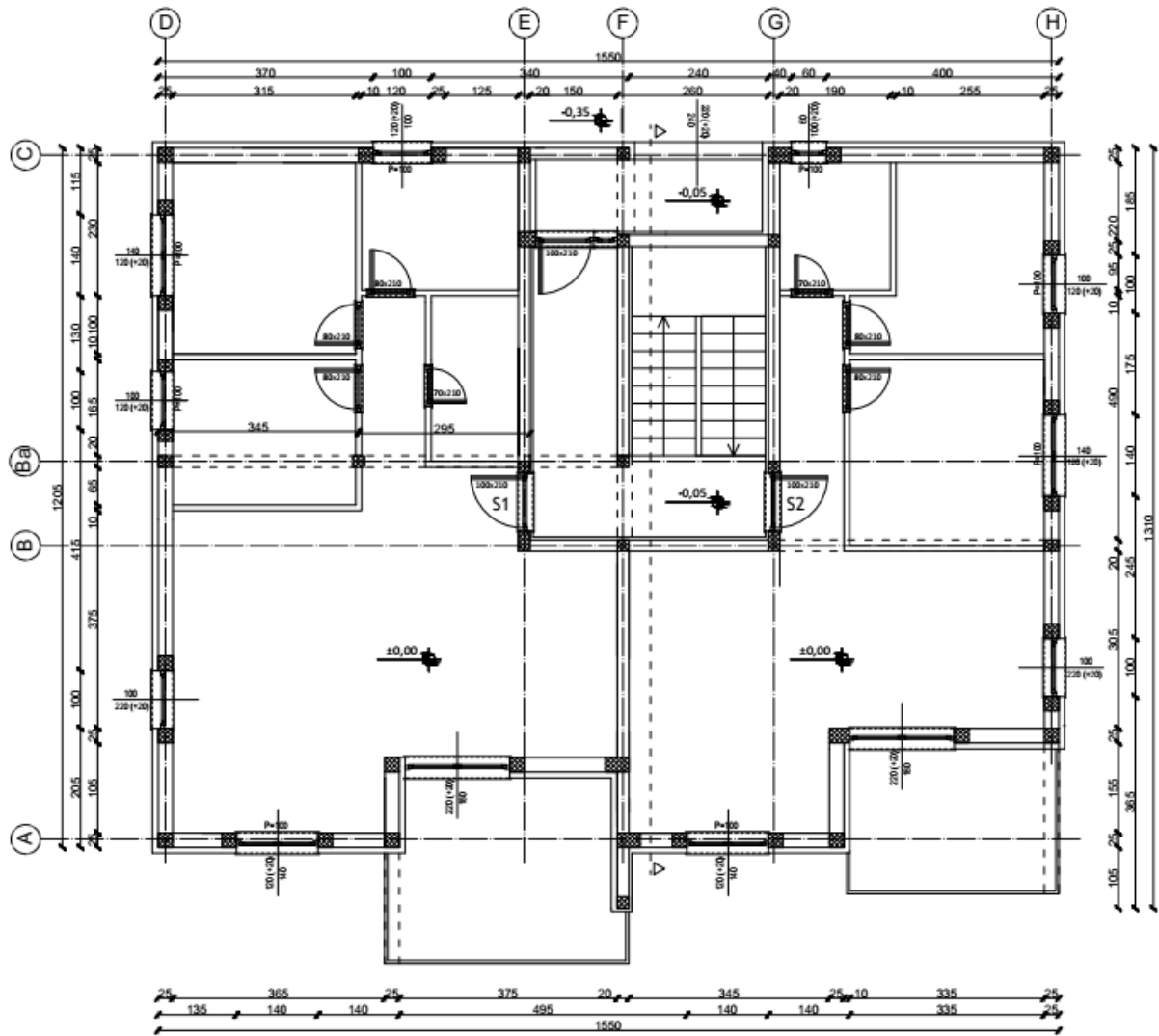
Slika 2: Tlocrt prizemlja
