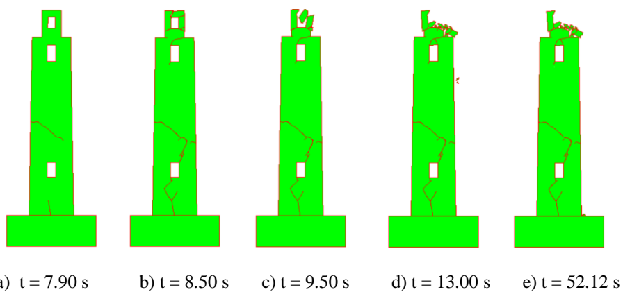
Slika 131. Širenje i nastanak pukotina za vršno ubrzanje a_g = 1.85 g za South Iceland
