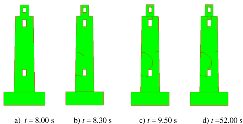
Slika 165. Širenje i nastanak pukotina za vršno ubrzanje \mathbf{a}_g = 1.00 \text{ g} za South Iceland
