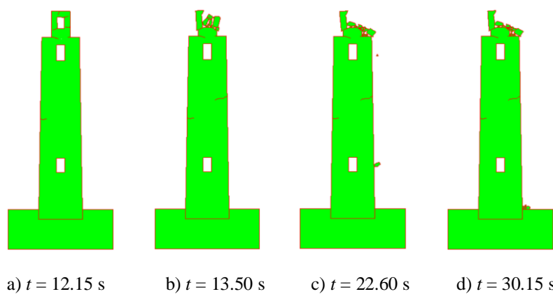
Slika 176. Širenje i nastanak pukotina za vršno ubrzanje a_g = 3.00 g za Campano Lucano
