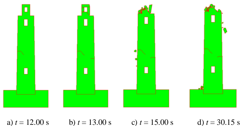
Slika 178. Širenje i nastanak pukotina za vršno ubrzanje a_g = 3.40 g za Campano Lucano
