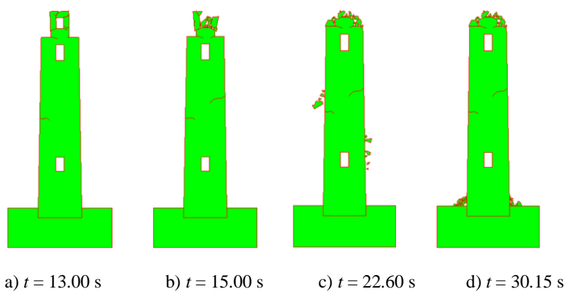
Slika 177. Širenje i nastanak pukotina za vršno ubrzanje a_g = 3.20 g za Campano Lucano
