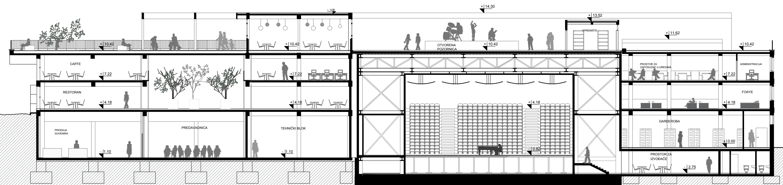
PRESJEK 2 - 2
