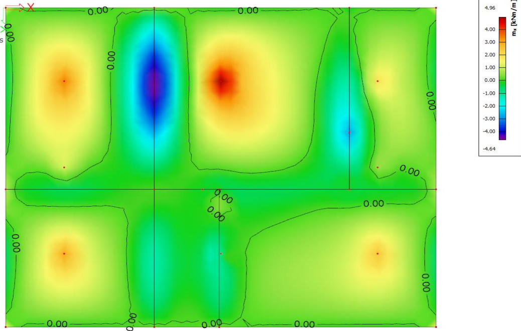
A_{S1,x} [cm^2/m']
