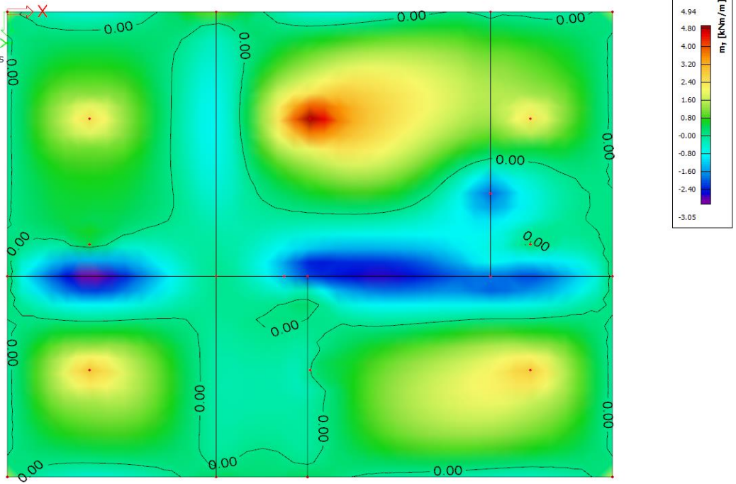
A_{S1,y} [cm^2/m']
