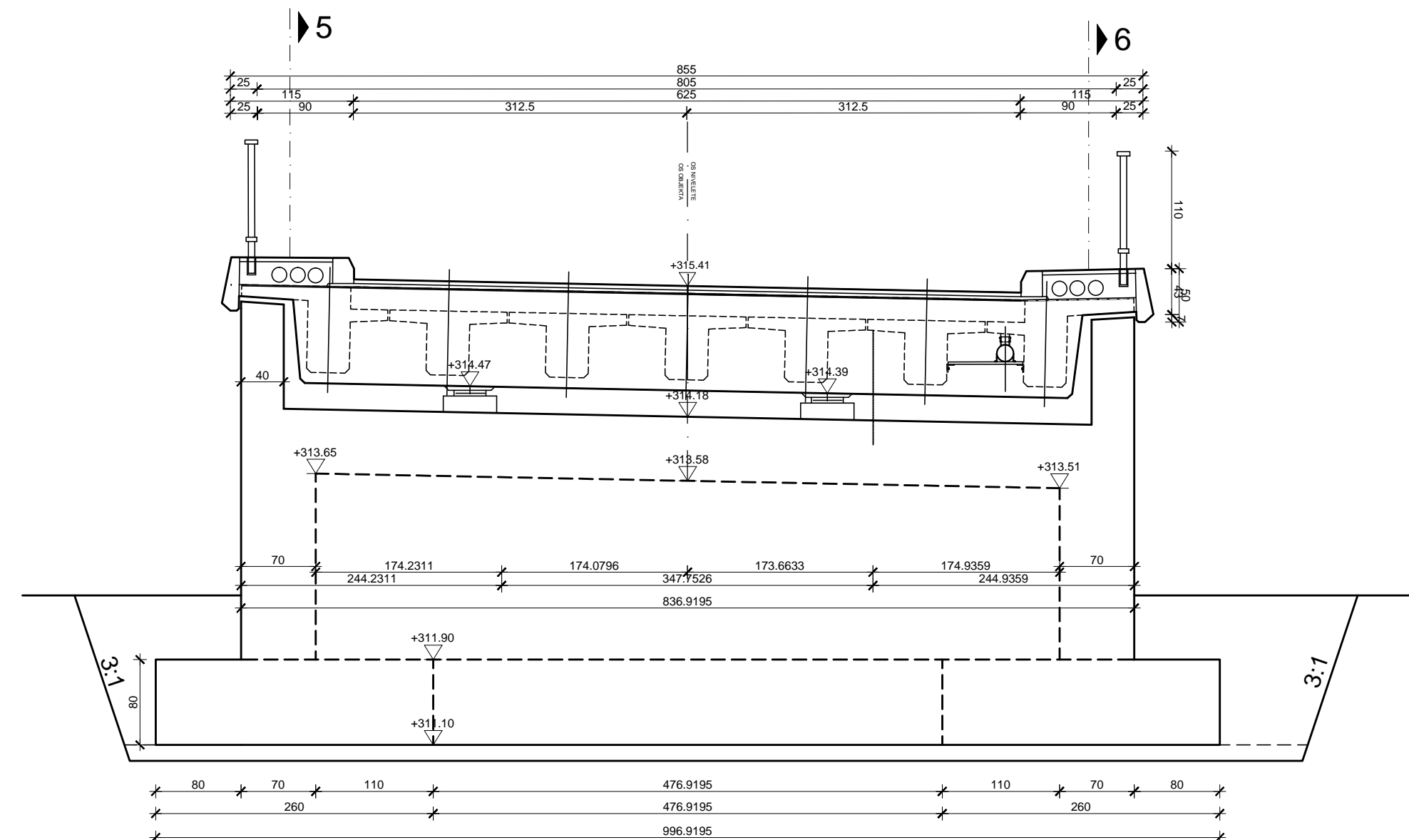
Presjek 1-1
