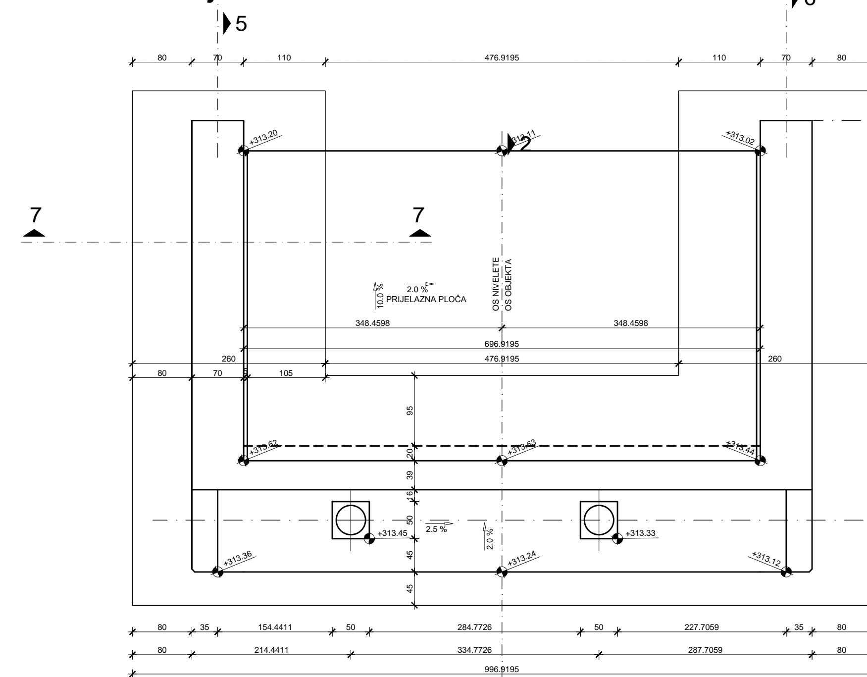
Presjek 4-4
