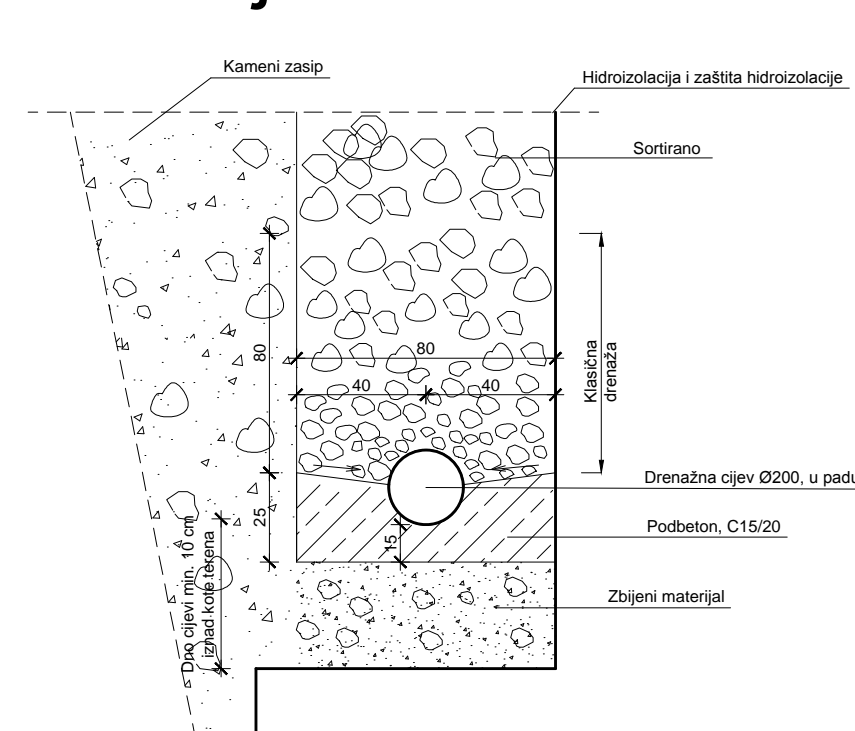
Detalj drenaže
