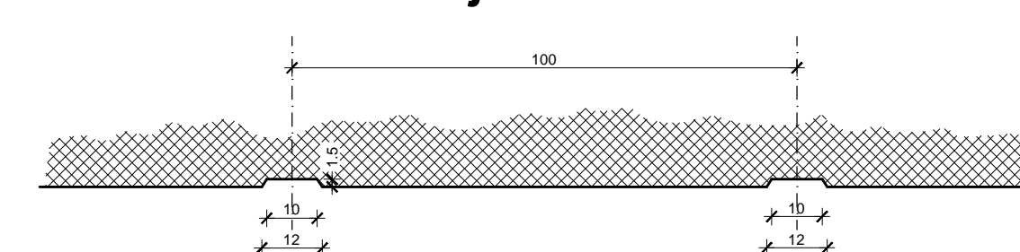
Detalj kanelura
