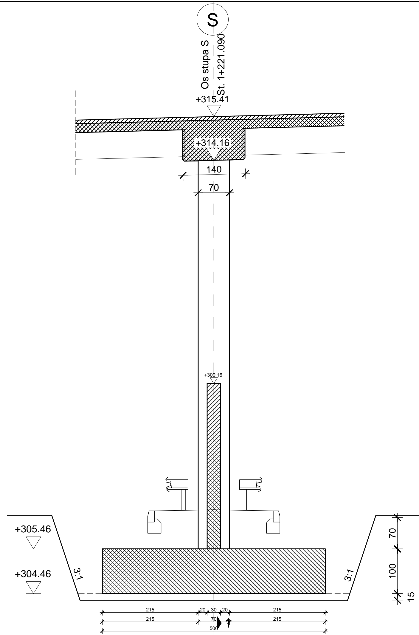
Presjek 3-3
