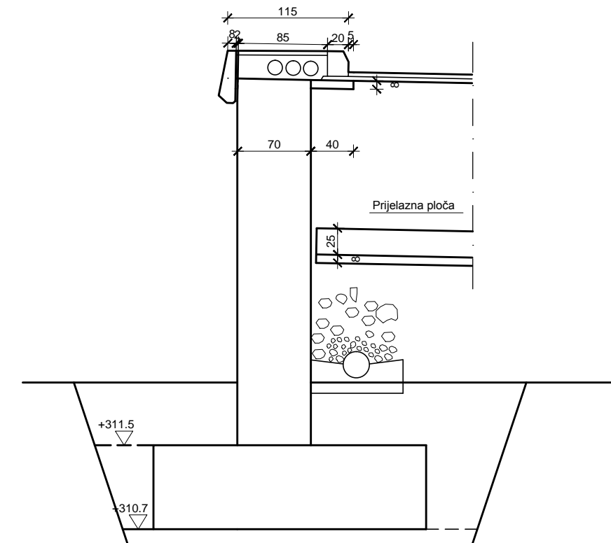
Presjek 7-7
