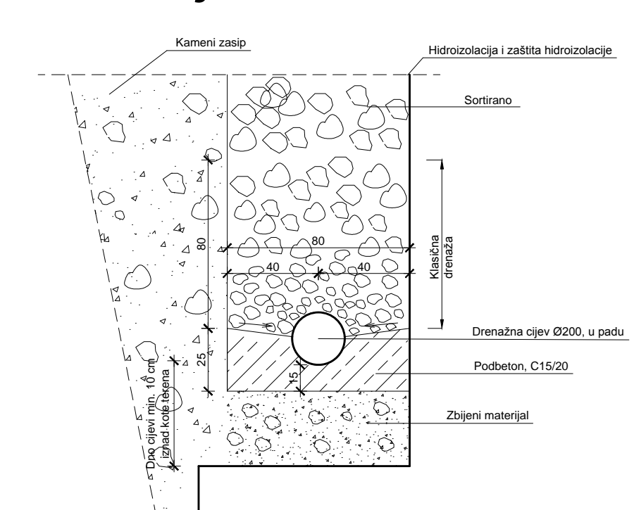
Detalj drenaže
