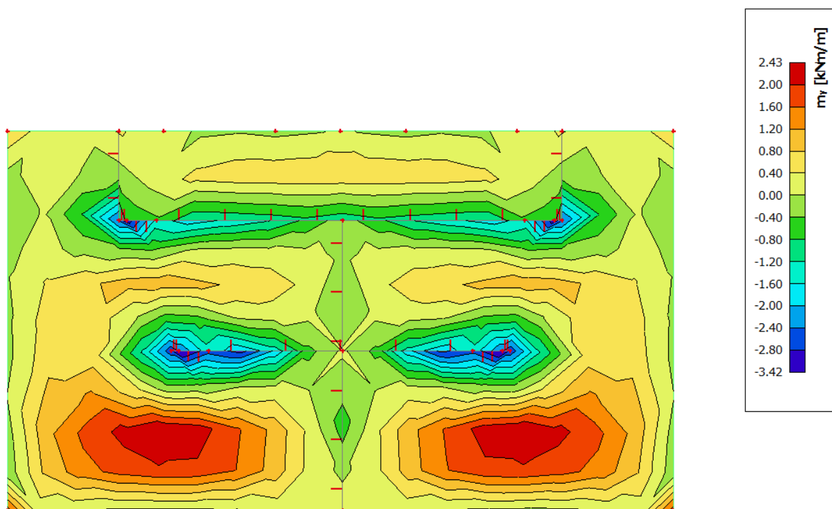
Slika 6.20 Potrebna površina armature A_s(cm^2/m) u y smjeru
