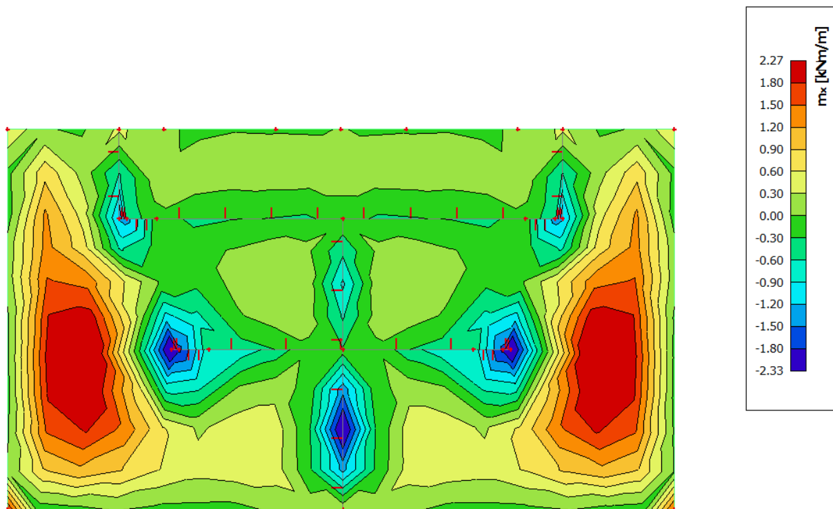
Slika 6.19 Potrebna površina armature A_s(cm^2/m) u x smjeru
