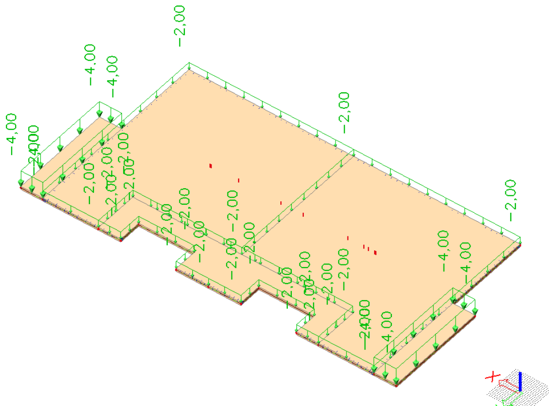
Slika 4.2.2 Promjenjivo djelovanje Q [ \text{kN/m}^2 ]
