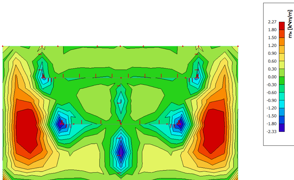
Slika 6.19 Potrebna površina armature A_s(\text{cm}^2/\text{m}) u x smjeru
