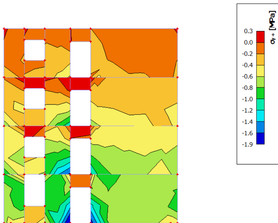
Slika 8.2.7 Naprezanja u zidu \sigma_y+ za kombinaciju GSN-1
