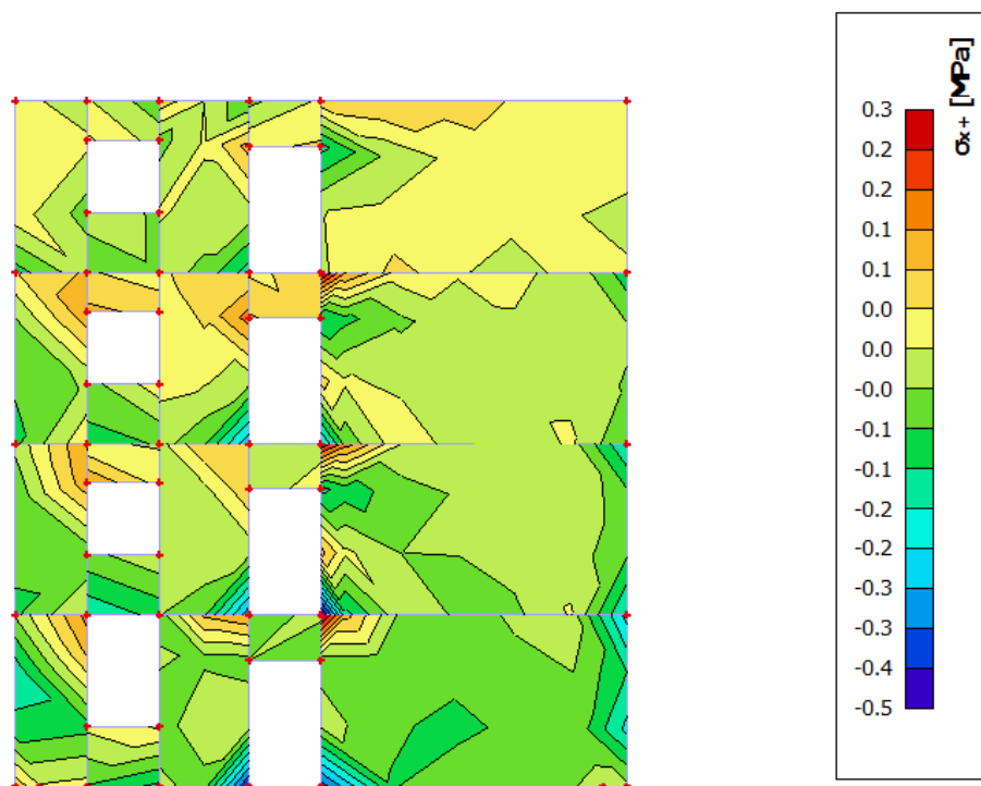
Slika 8.2.5 Naprezanja u zidu \sigma_{x+} za kombinaciju GSN-1
