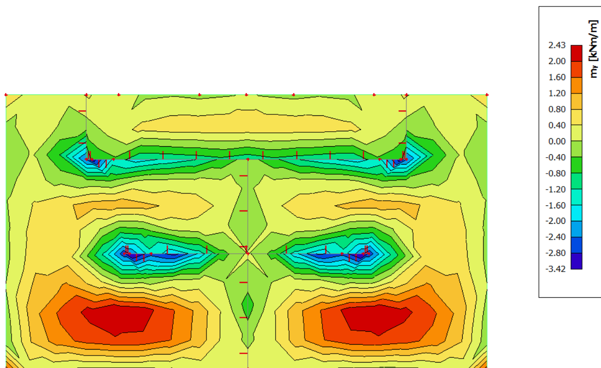
Slika 6.20 Potrebna površina armature A_s(\text{cm}^2/\text{m}) u y smjeru
