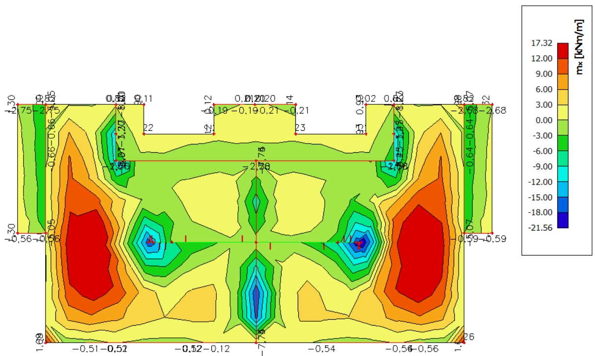
Slika 6.2 Moment savijanja M_{Ed,x} ( \text{kNm/m} ) za GSN-1
