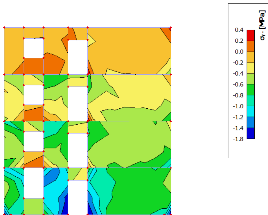
Slika 8.2.8 Naprezanja u zidu \sigma_y- za kombinaciju GSN-1
