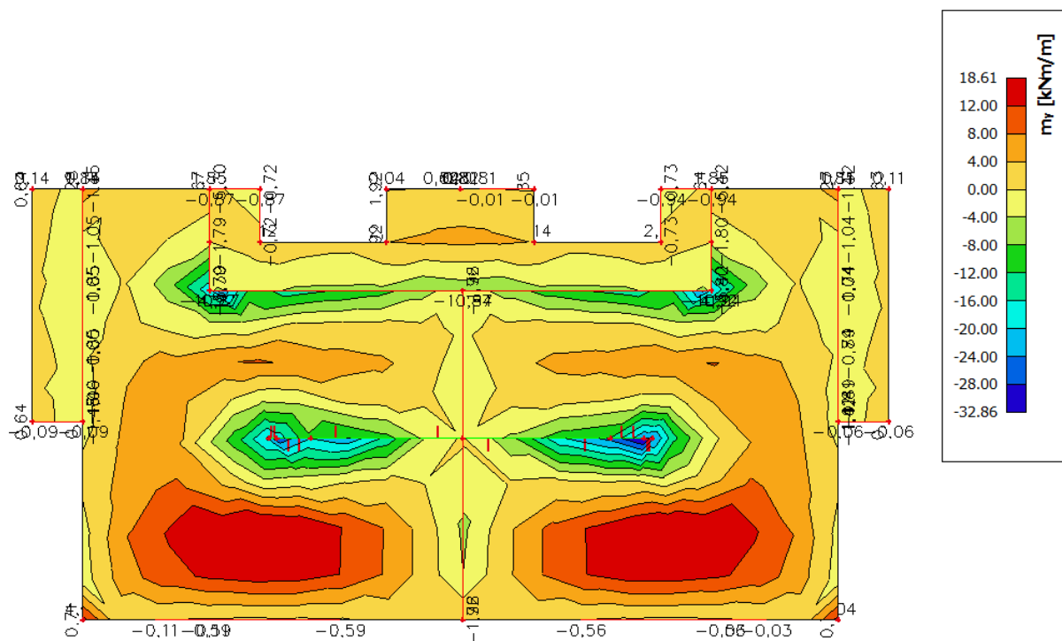
Slika 6.3 Moment savijanja M_{Ed,y} (kNm/m) za GSN-1
