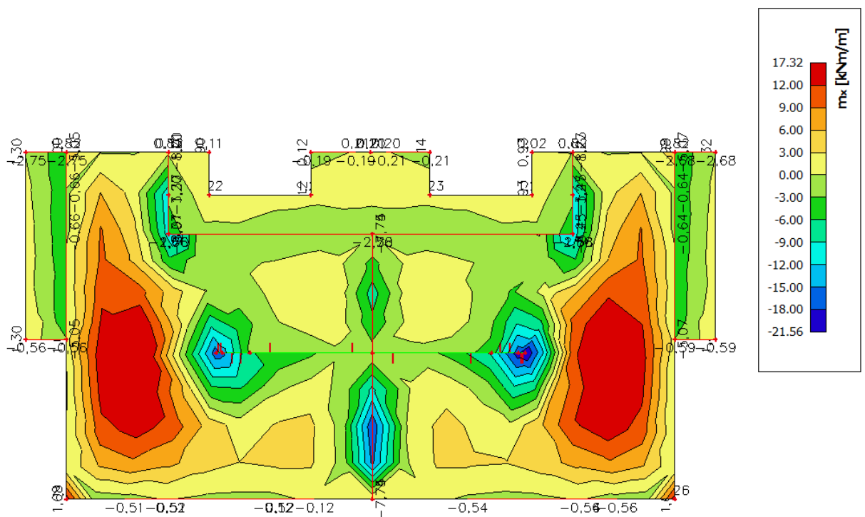
Slika 6.2 Moment savijanja M_{Ed,x} (kNm/m) za GSN-1
