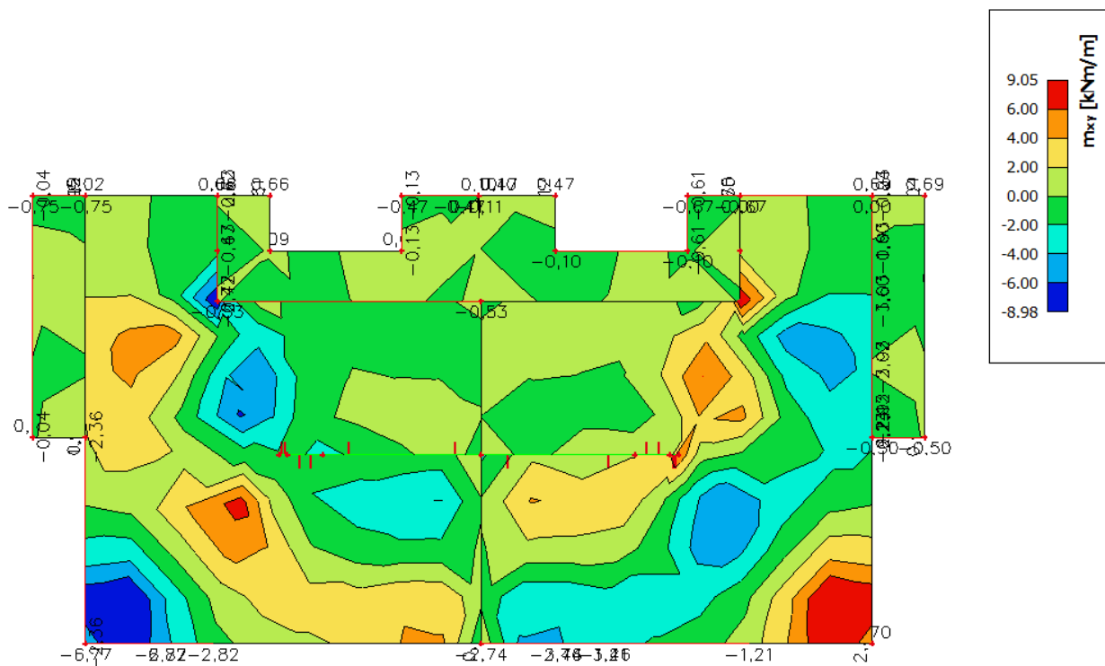
Slika 6.4 Moment savijanja M_{Ed,xy} (kNm/m) za GSN-1
