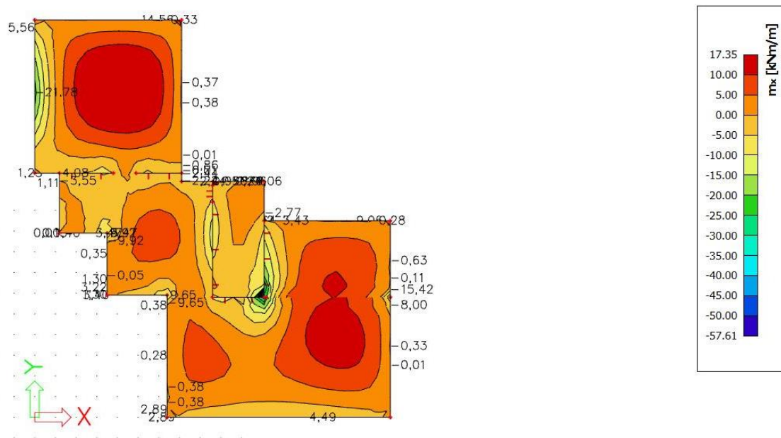
Slika 6.23 Moment savijanja M_{Ed,x} (kNm/m) za GSU-1
