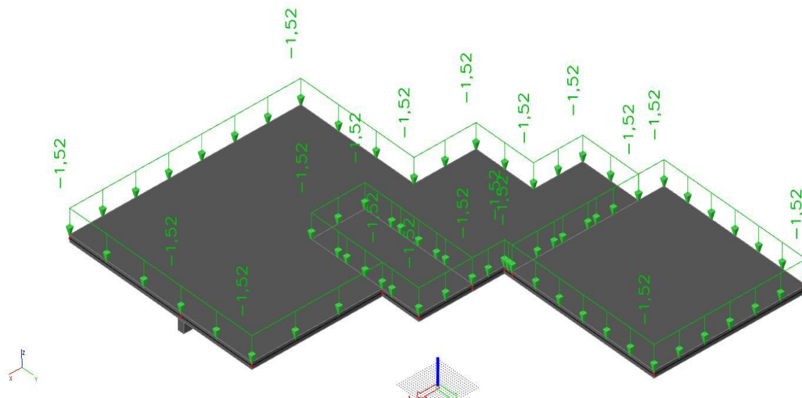
Slika 4.1.1 Dodatno stalno djelovanje G1 [ \text{kN/m}^2 ]
