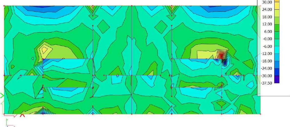
Slika 5.18 Poprečne sile V_{Ed,y} (kN/m) za GSN-1
