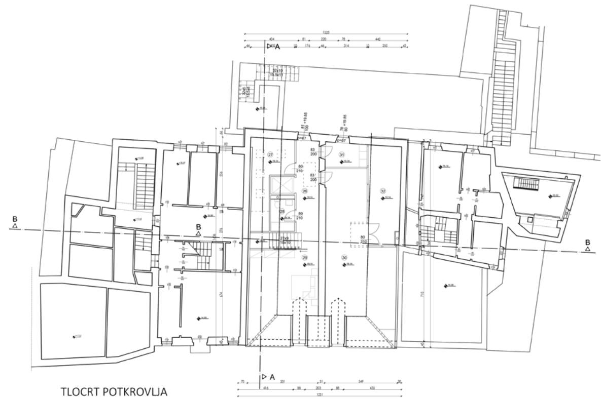
TLOCRT PRIZEMLJA
