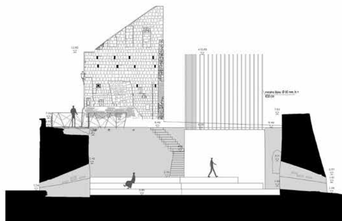
presjek 1-1
