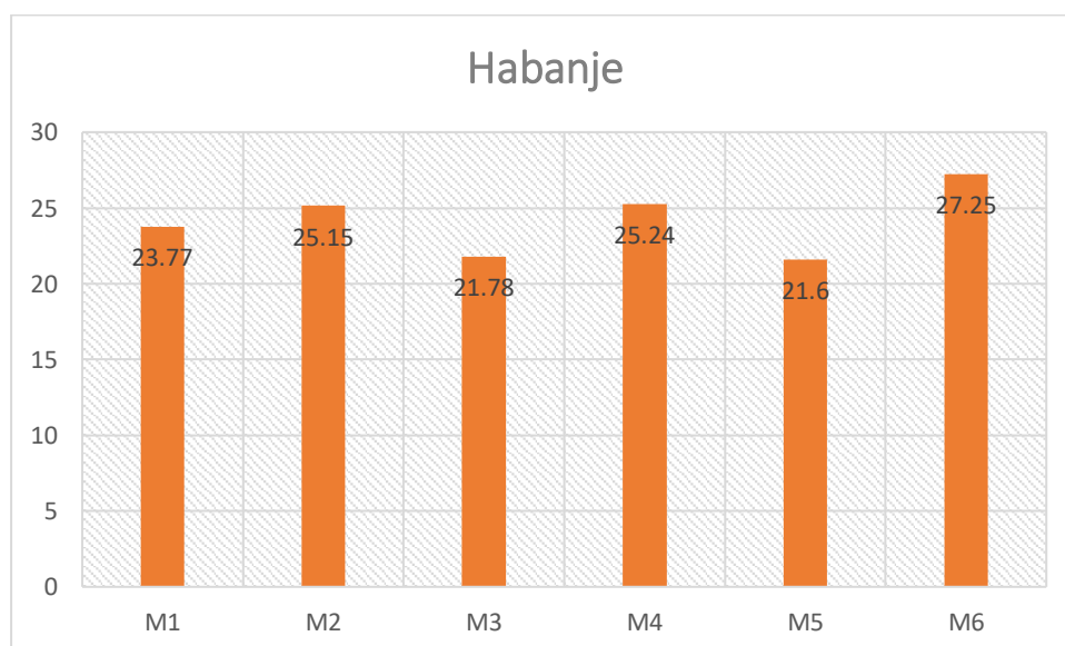
Graf 3.5.3.1. Otpornost na habanje svih ispitanih uzoraka
