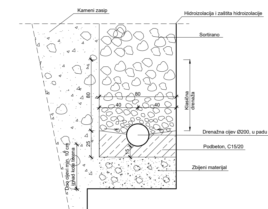
Detalj drenaže
