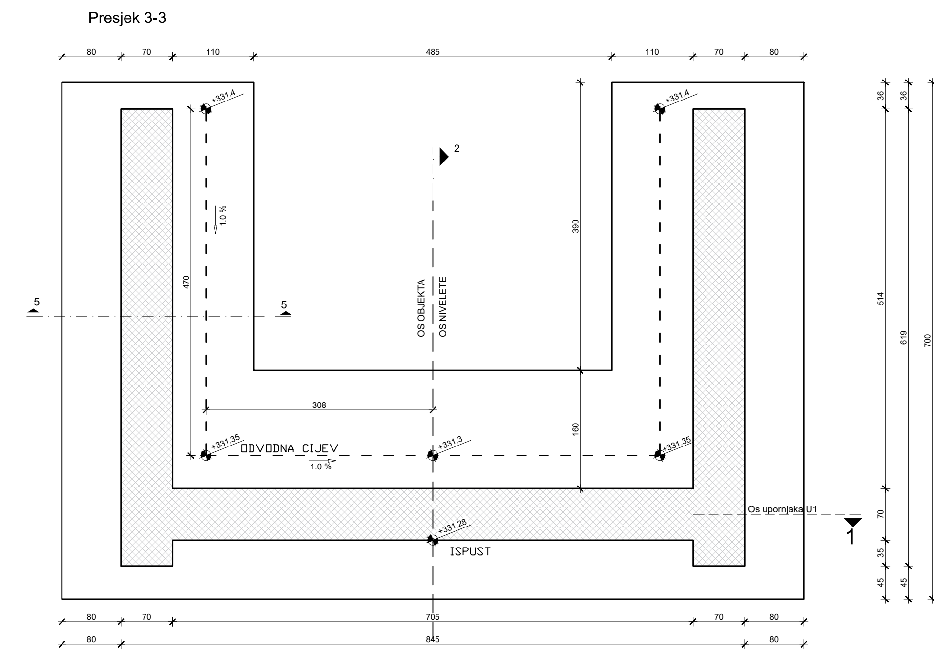
Presjek 3-3
