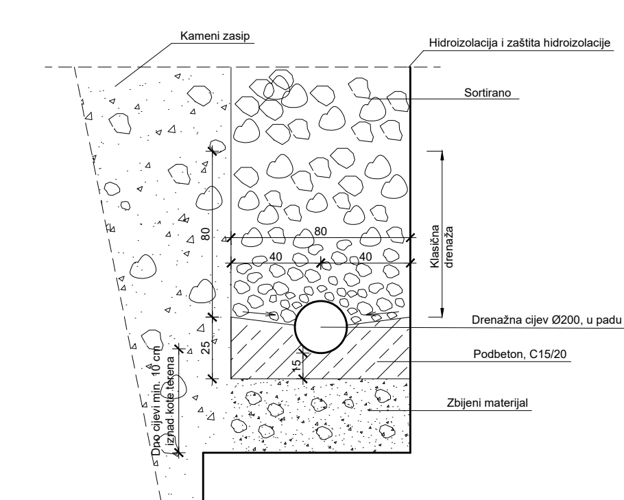
Detalj drenaže
