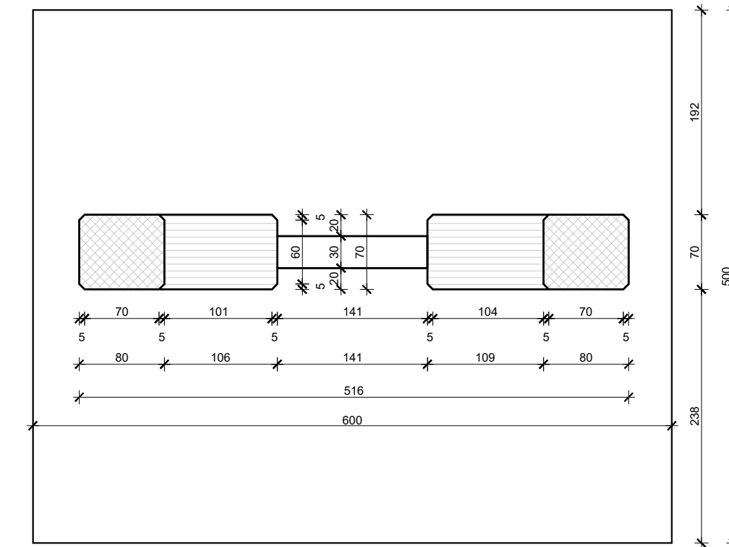
Presjek 3-3
