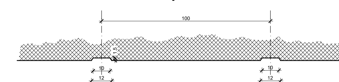
Detalj kanelura
