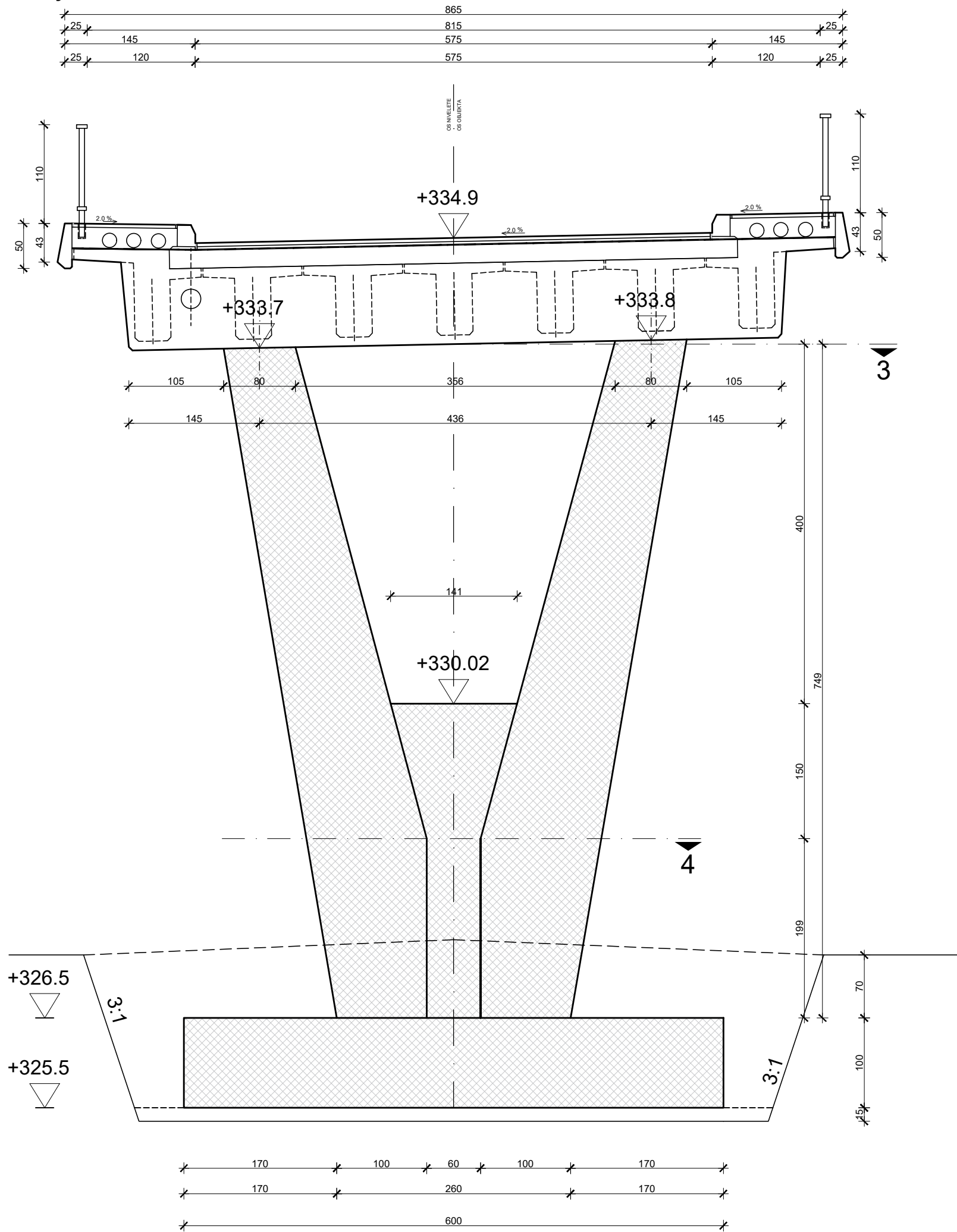
Presjek 1-1
