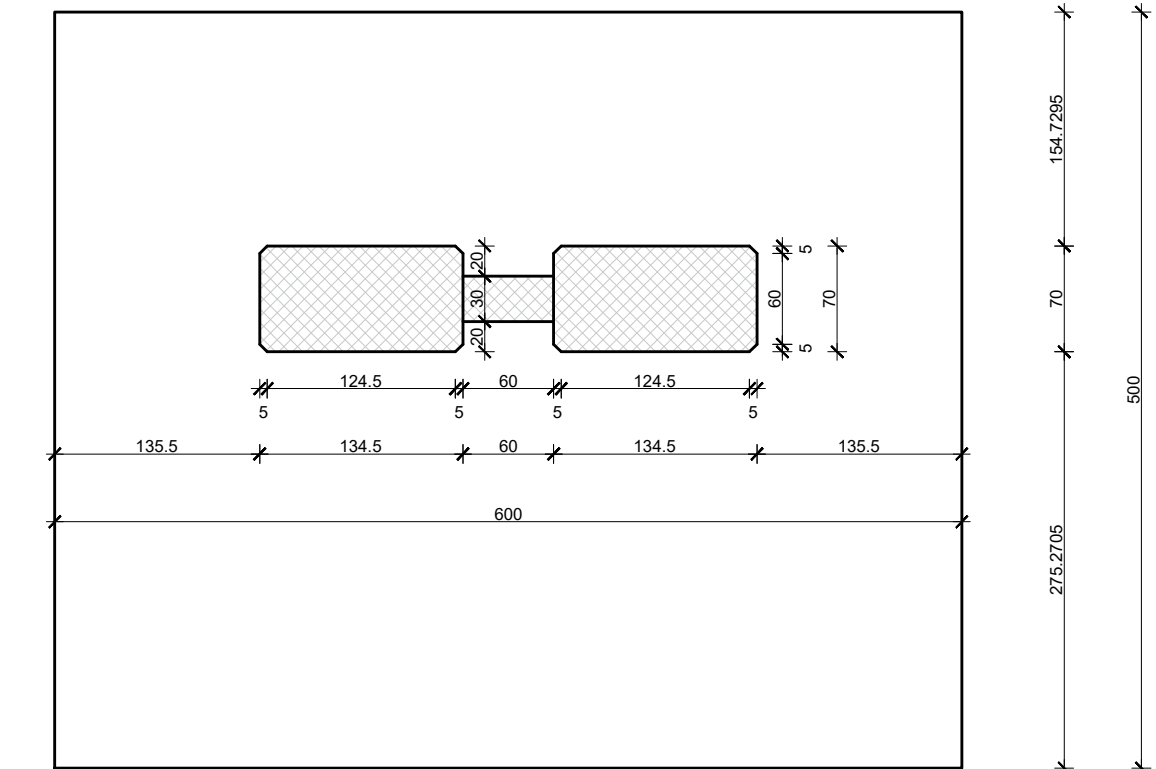
Presjek 4-4
