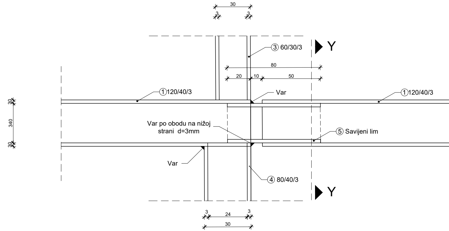
Detalj D 2 1:2
