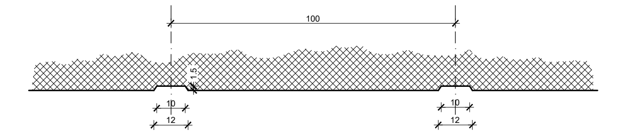
Detalj kanelura
