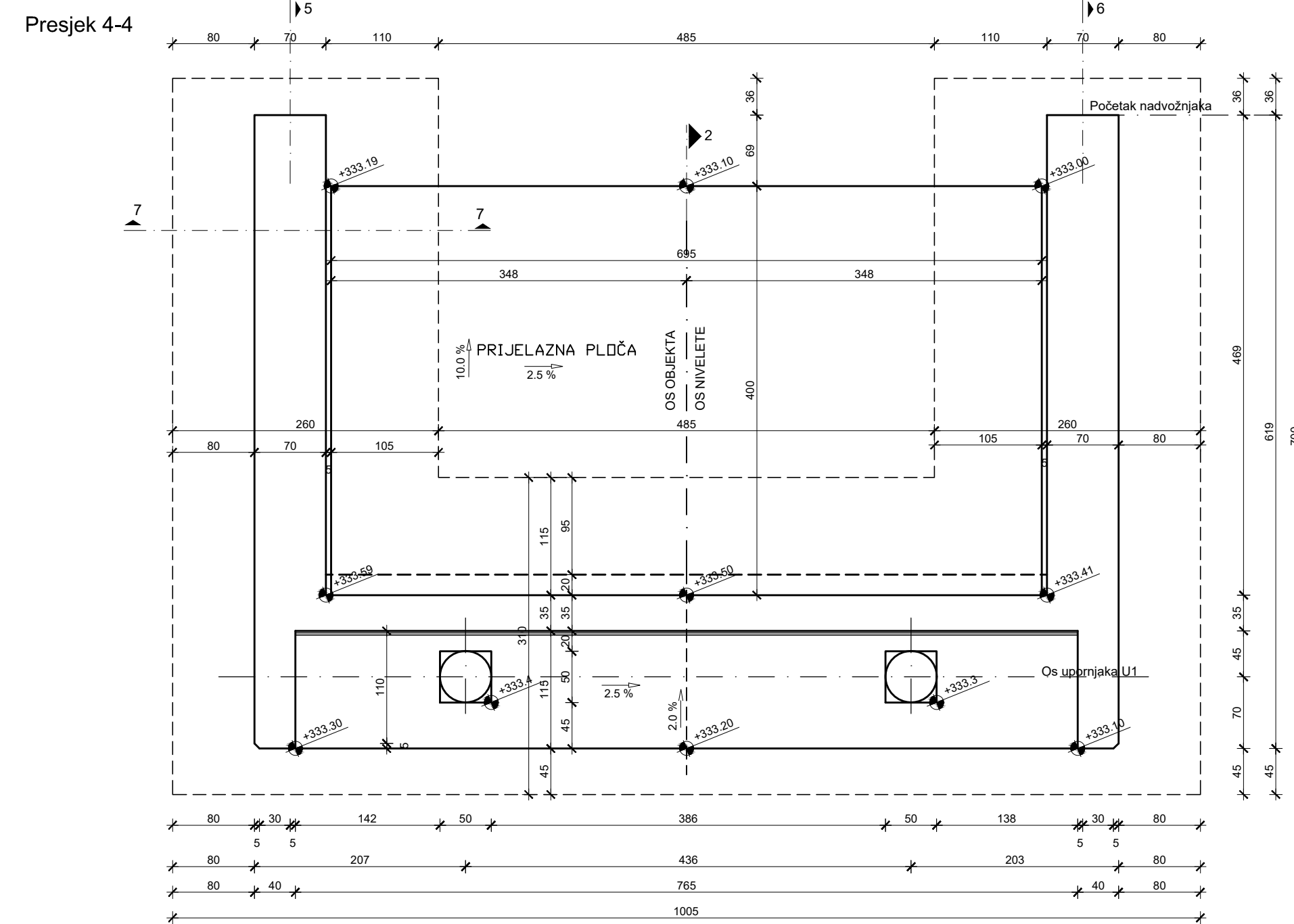
Presjek 4-4
