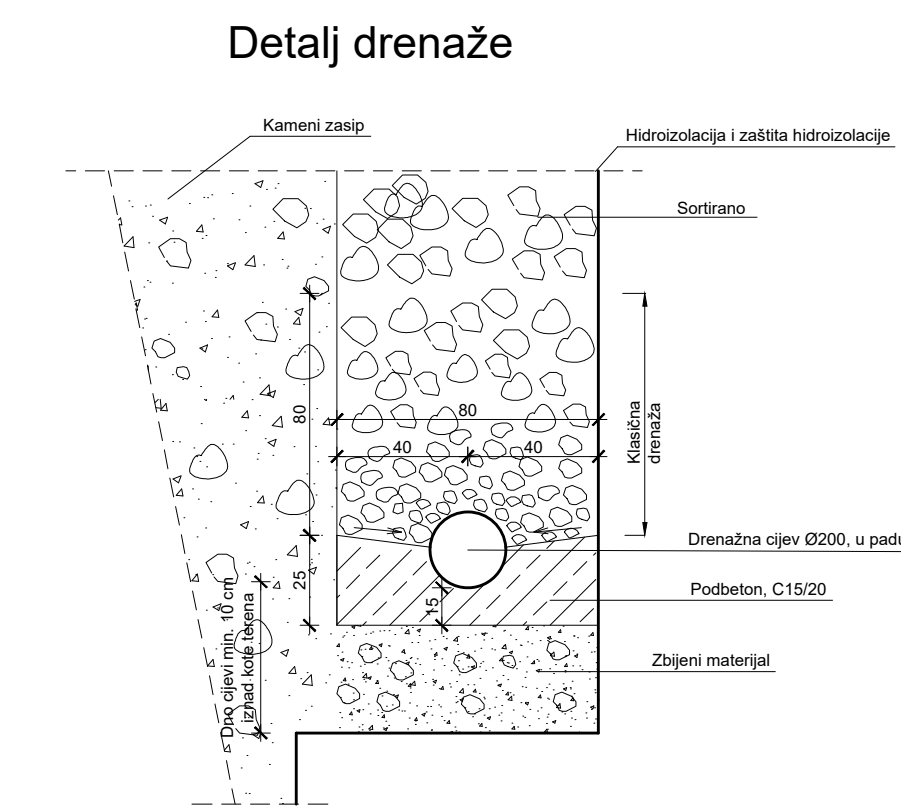
Detalj drenaže
