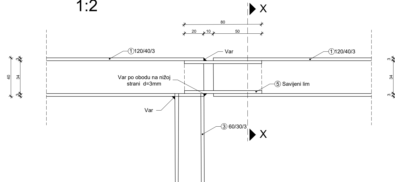
Detalj D 2 1:2
