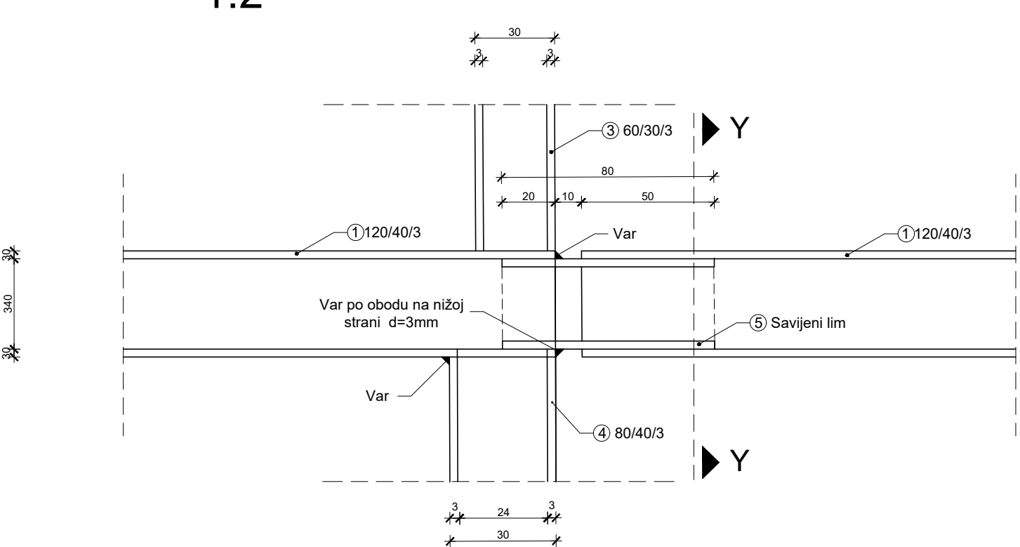
Detalj D 2 1:2
