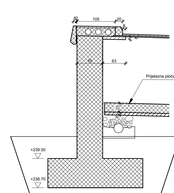
Presjek 7-7
