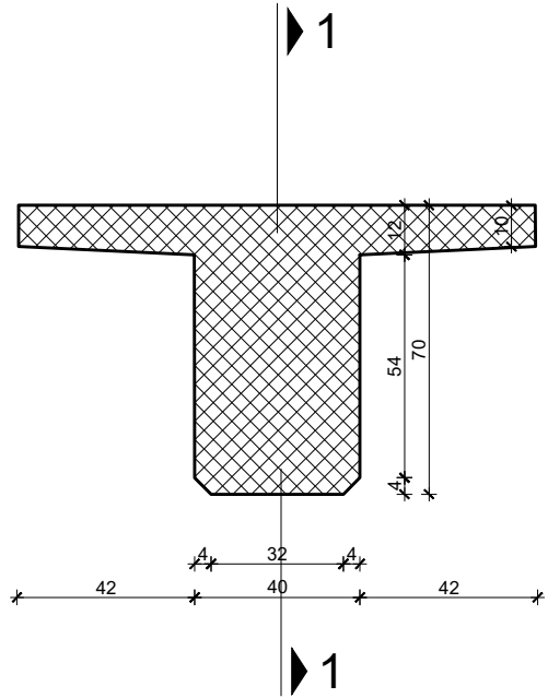
Presjek 3-3
