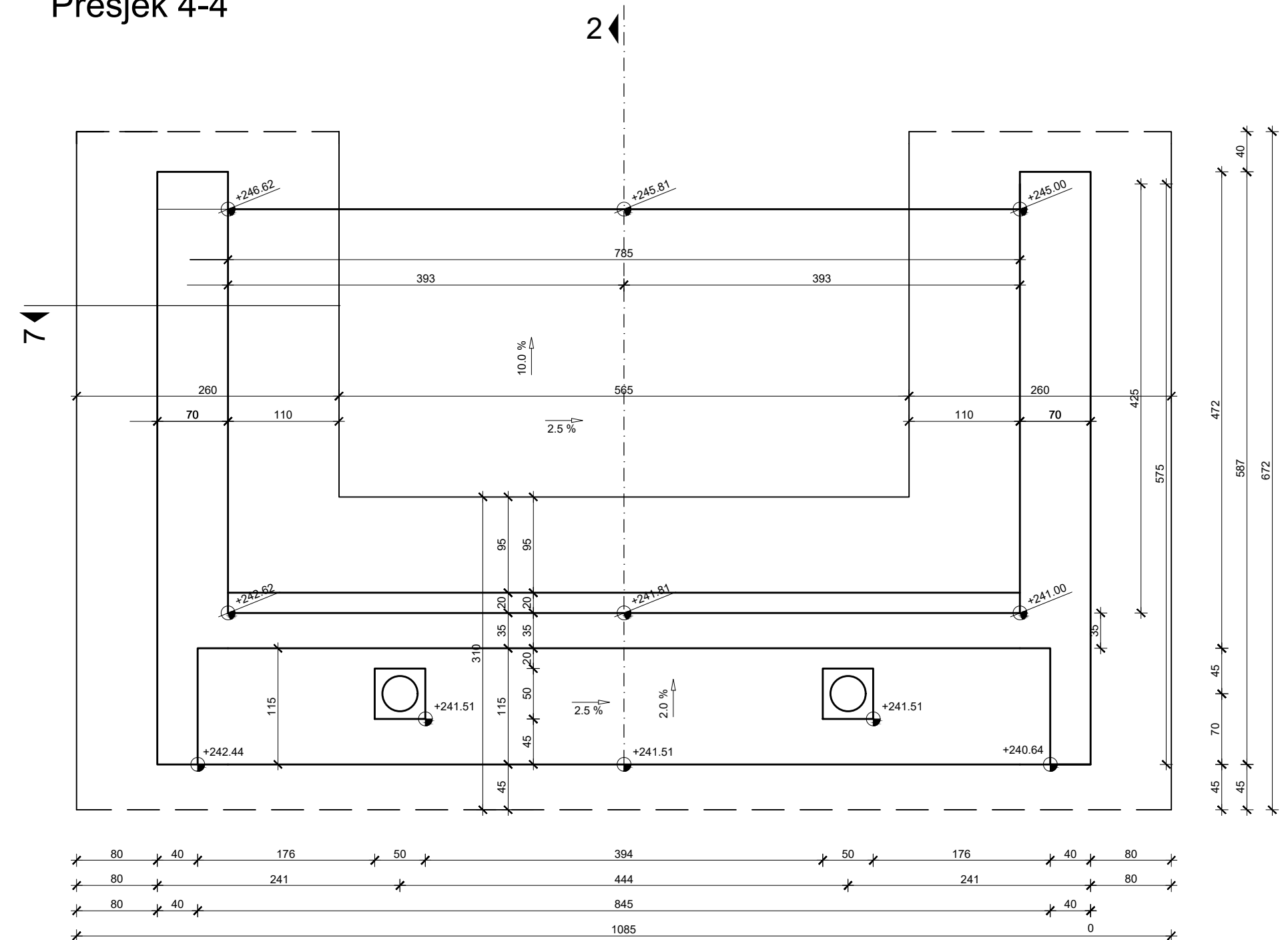
Presjek 4-4
