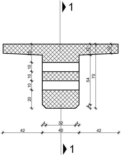
Presjek 2-2
