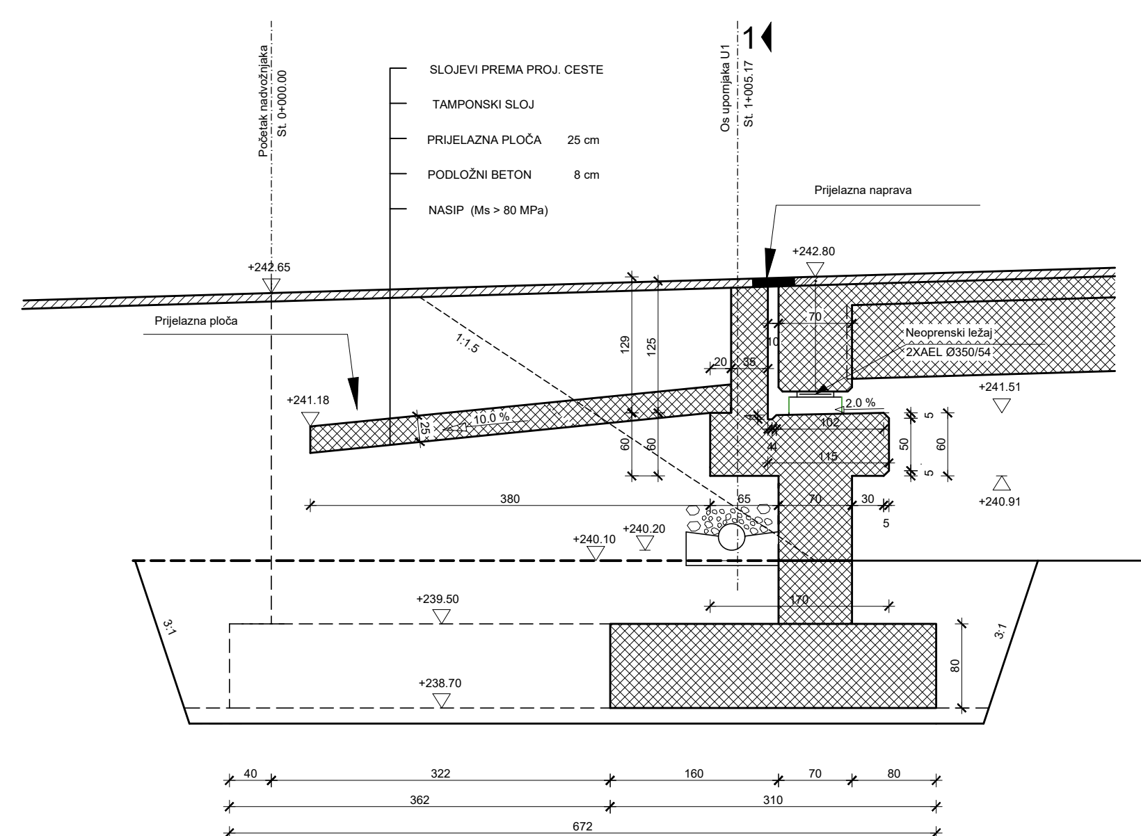
Presjek 3-3
