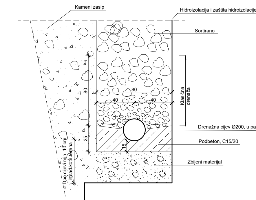
Detalj drenaže
