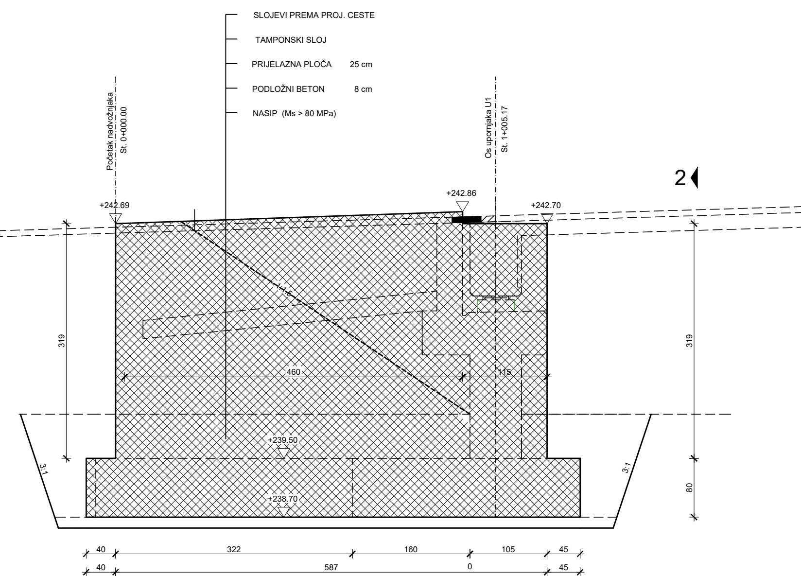
Presjek 5-5
