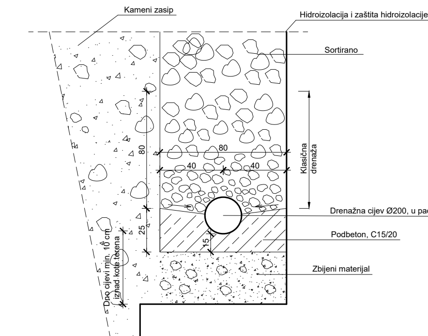
DETALJ DRENAŽE
