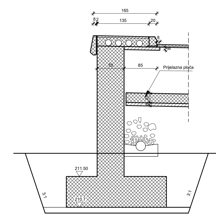
PRESJEK 7-7
