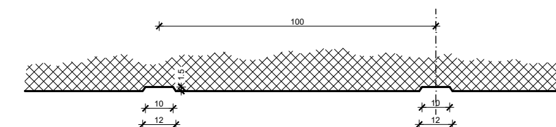
Detalj drenaže
