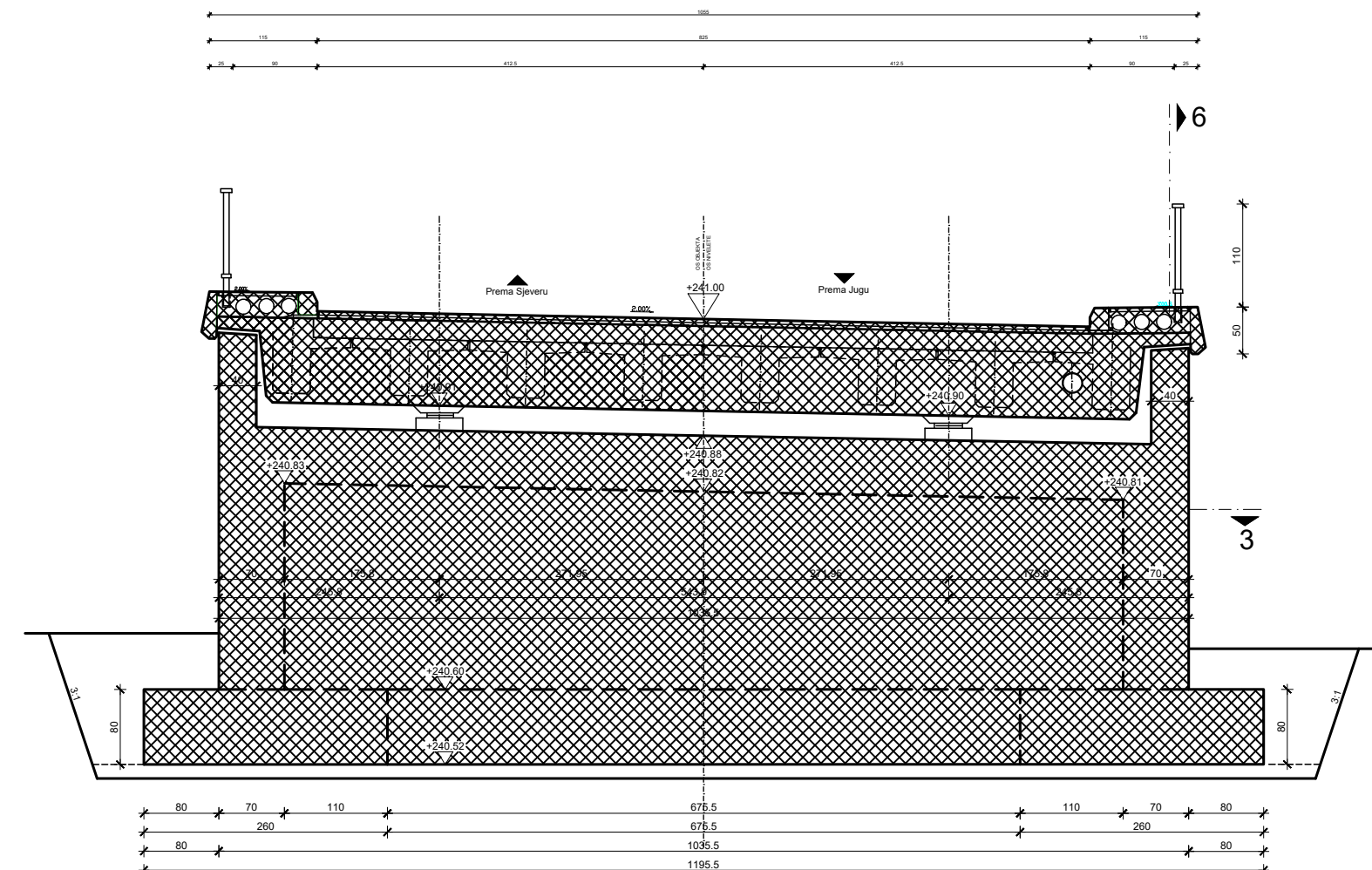
Presjek 4-4
