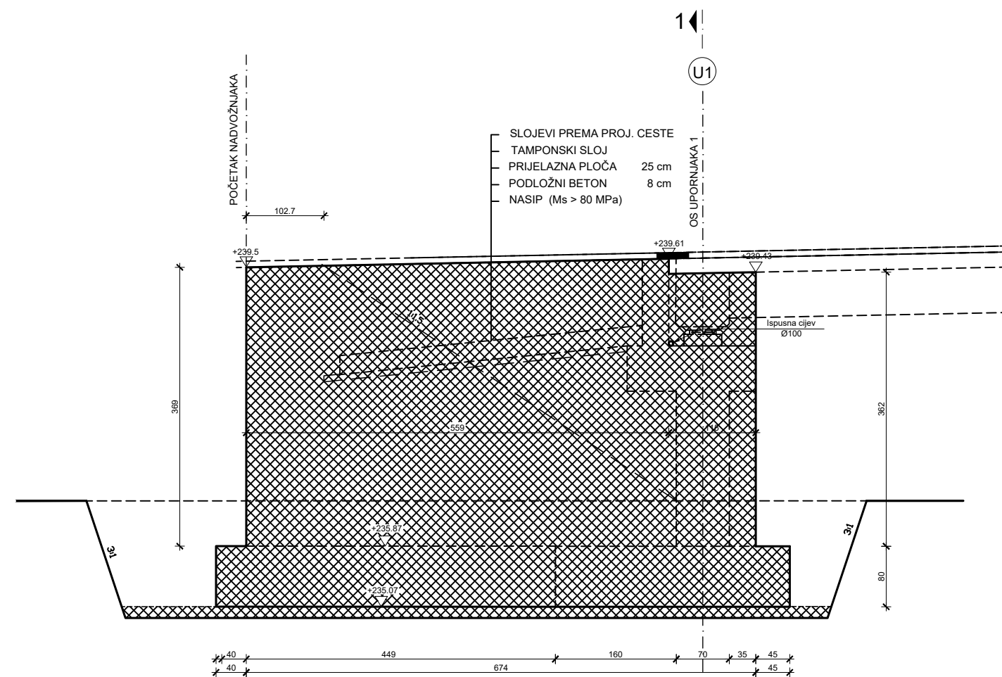
Presjek 6-6
