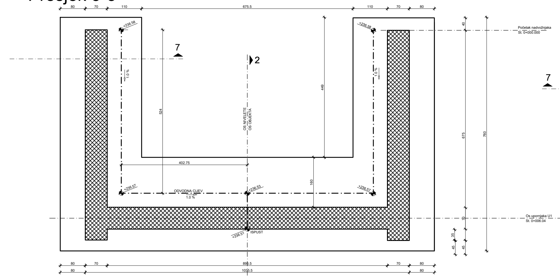
Presjek 3-3
