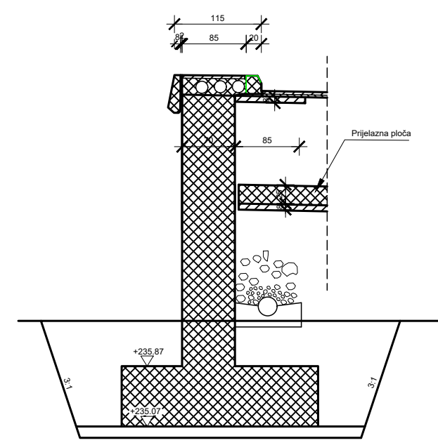
Detalj drenaže
