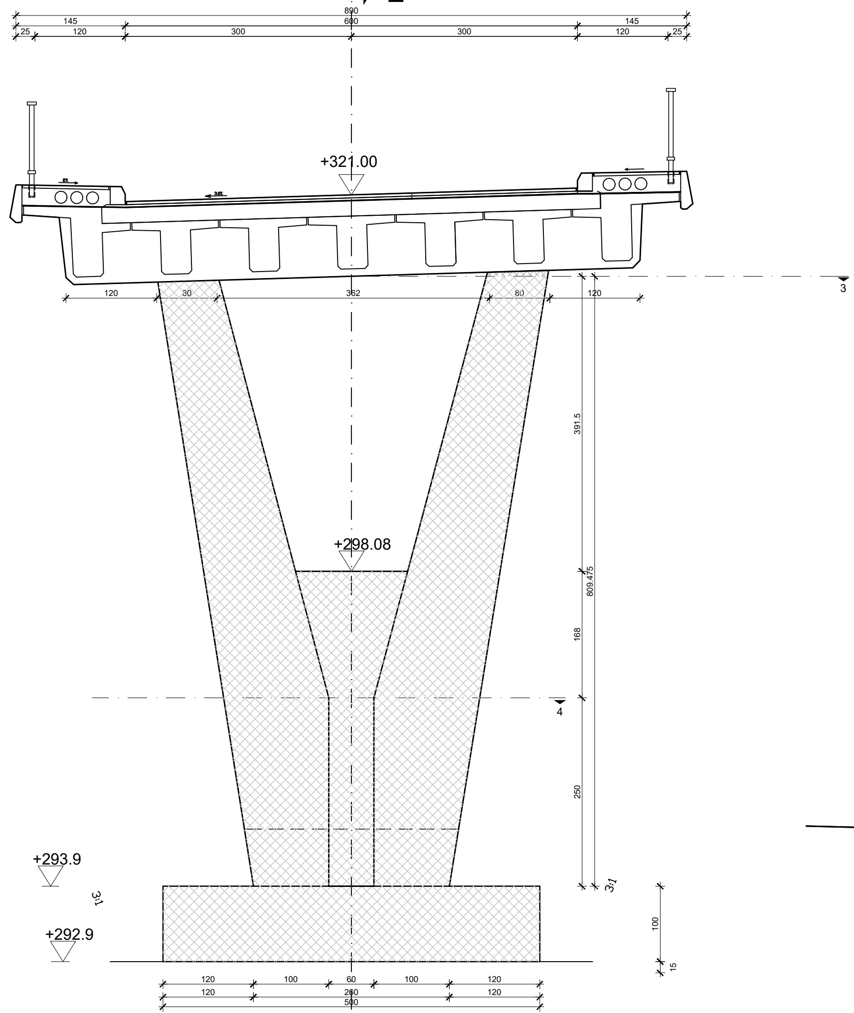
Presjek 1-1
