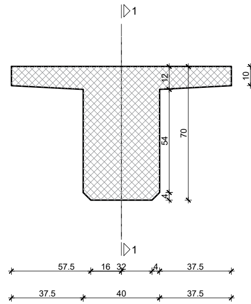
Presjek 2-2
