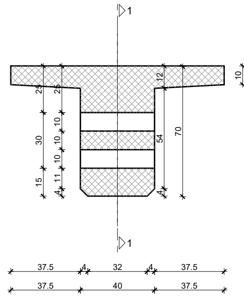
Presjek 3-3
