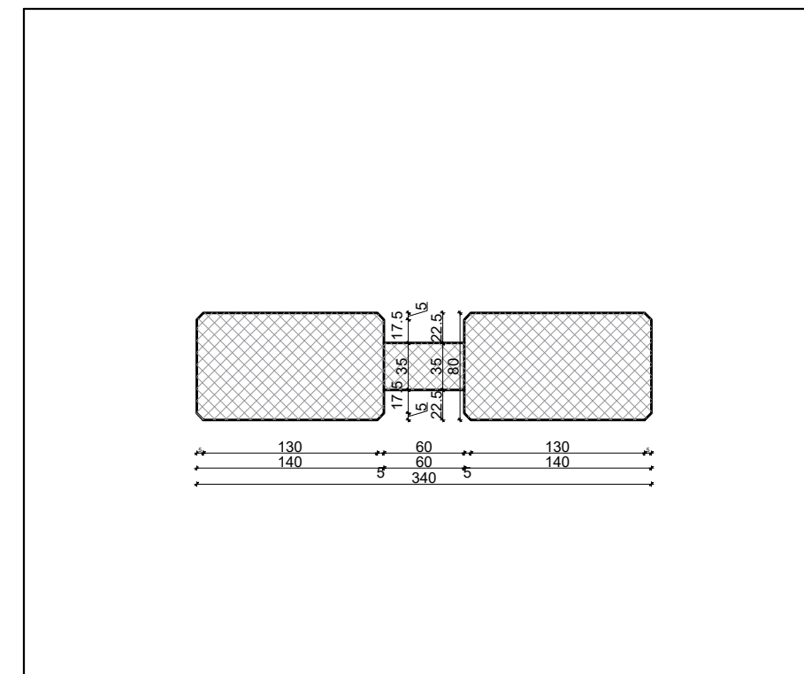
Presjek 4-4
