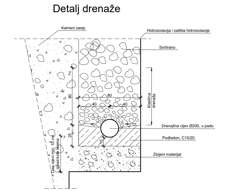
Detalj drenaže
