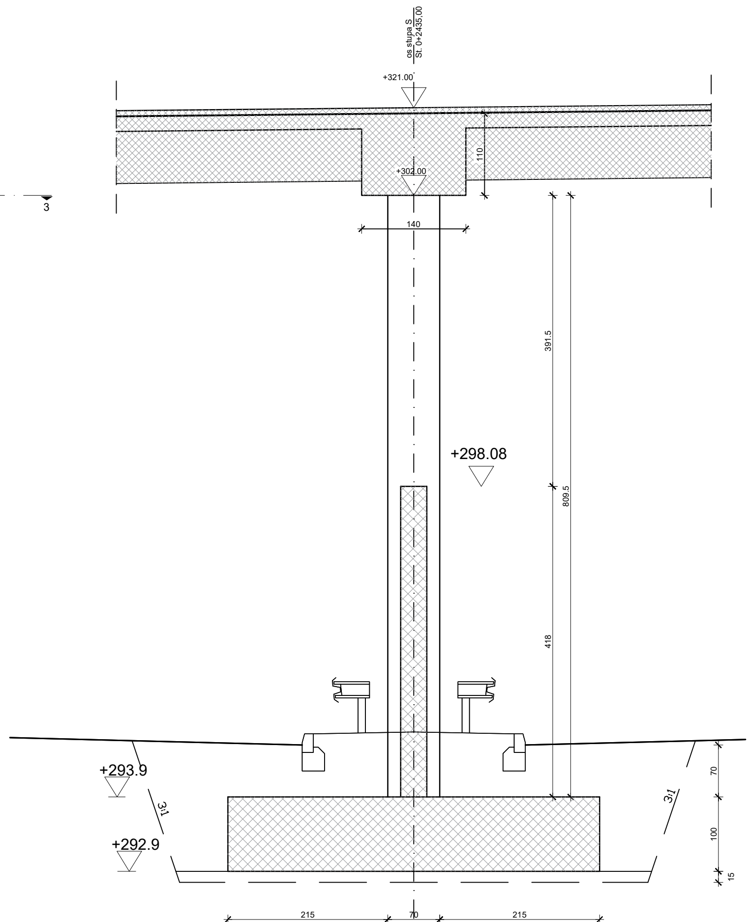
Presjek 2-2
