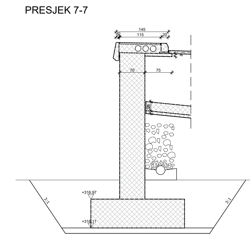
PRESJEK 7-7
