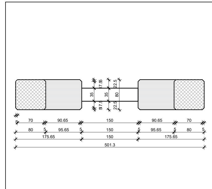
Presjek 3-3
