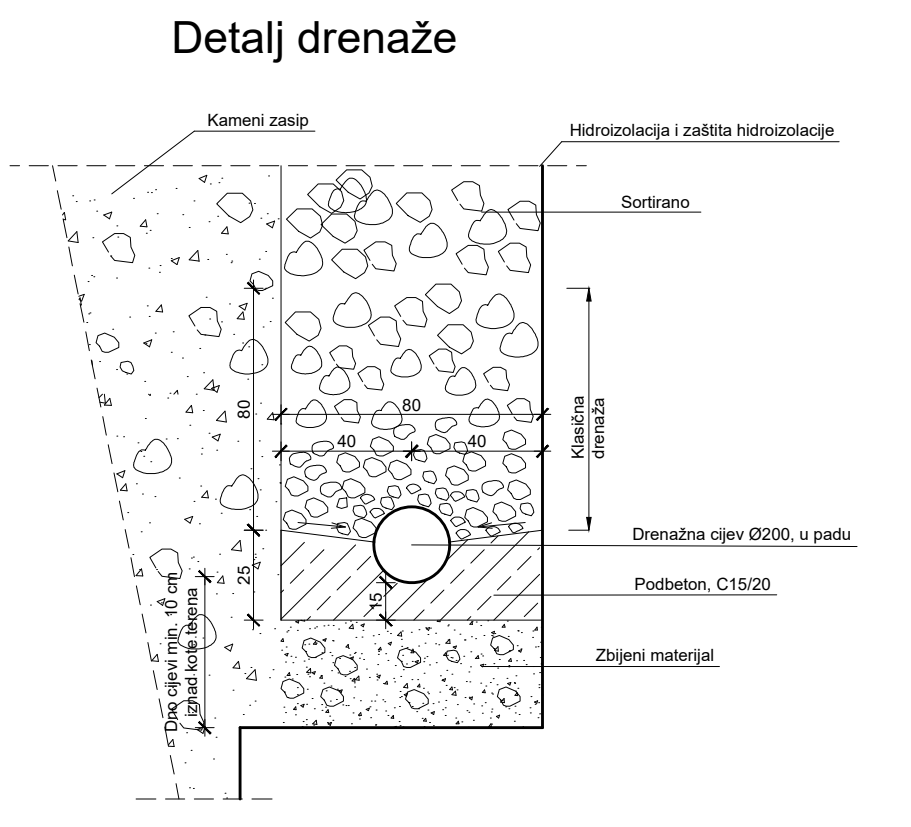
Detalj kanelura
