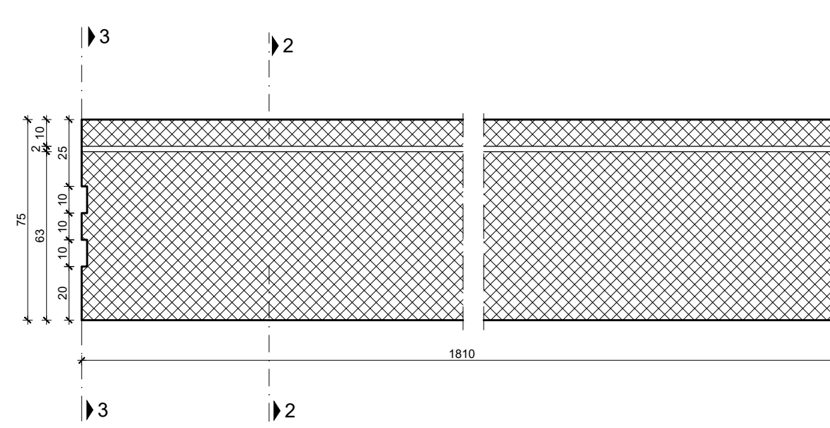
Presjek 1-1
