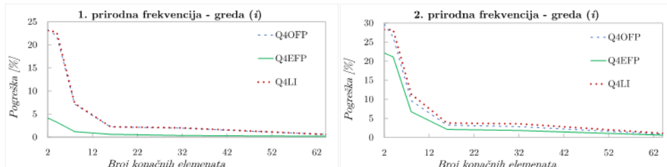
Slika 1. Konvergenzijska studija rezultata prvih dviju prirodnih frekvencija konzolne ravninske gređe ( i ) diskretizirane Q4 elementima
