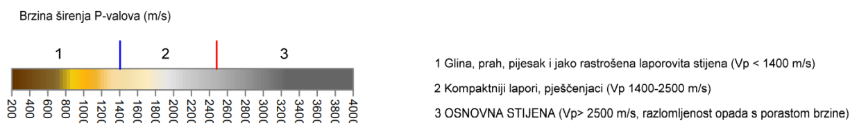
Slika 9. Klasifikacija tla i stijenovite mase ovisno o brzini P-valova (Nearest neighbour interpolacija) [3]
