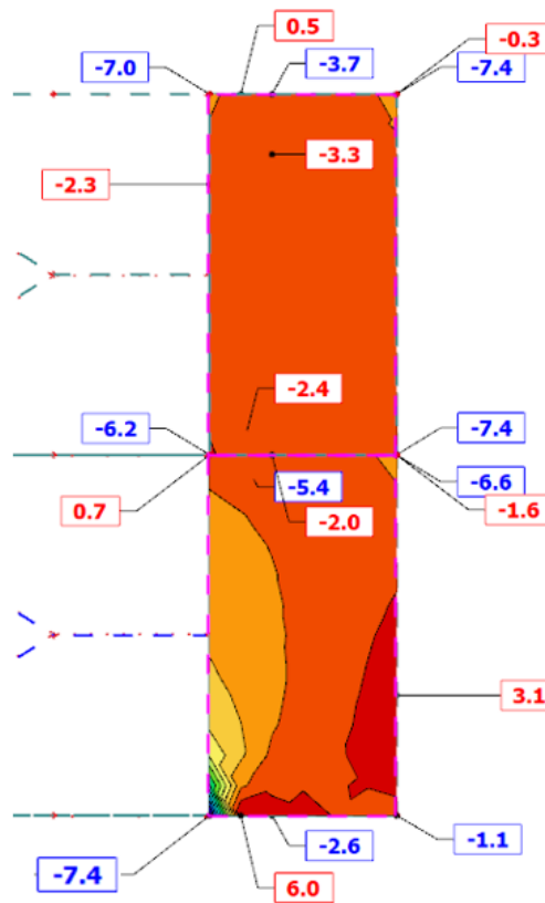
Slika 11.17. Prikaz glavnih naprezanja \sigma_x za visokostijeni nosač
