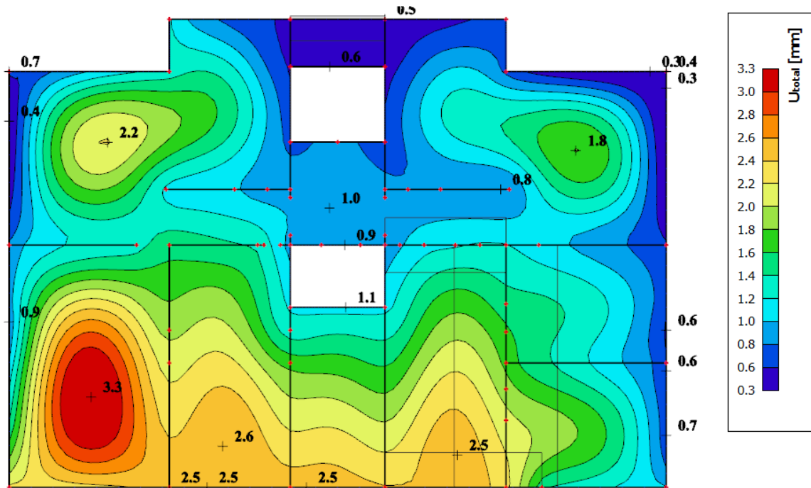
Slika 10.164. Prikaz progiba za ploču za kombinaciju GSU
