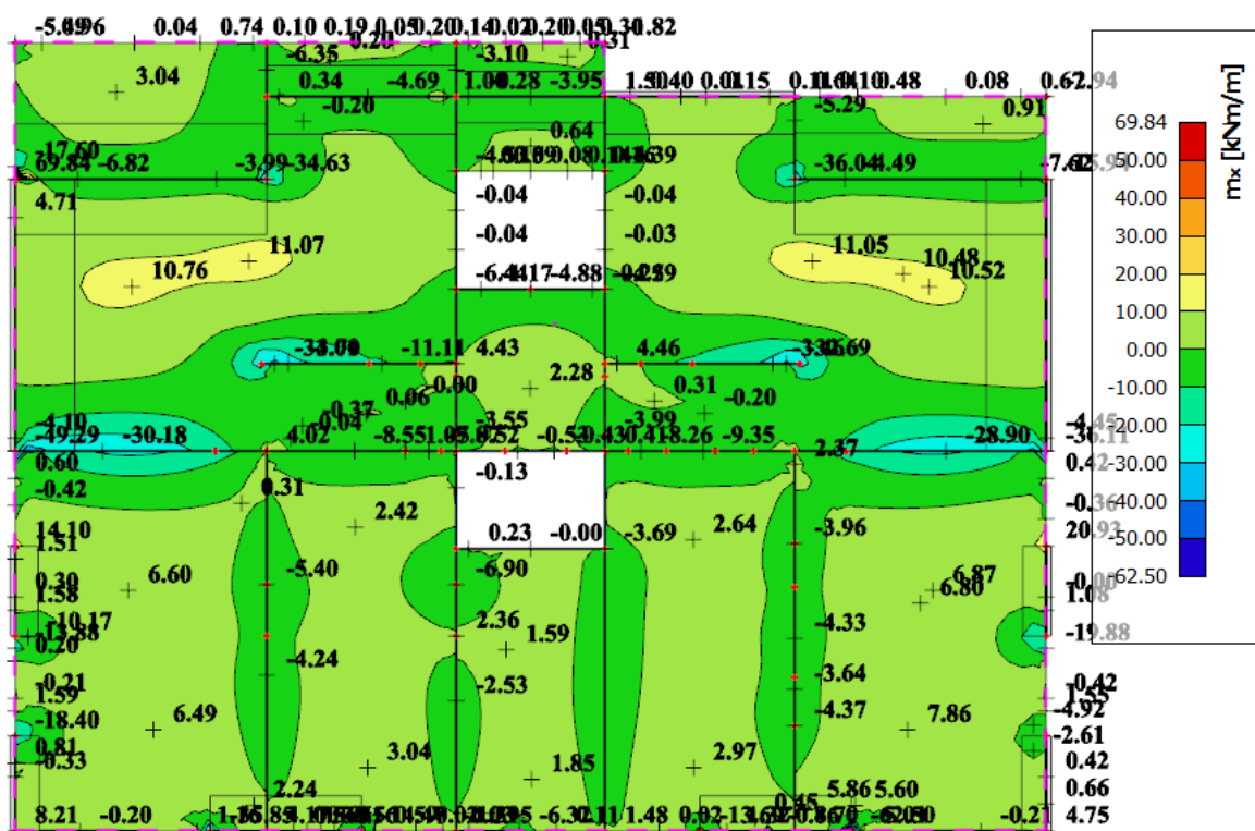
Slika 10.89. Prikaz momenata savijanja - m_x
