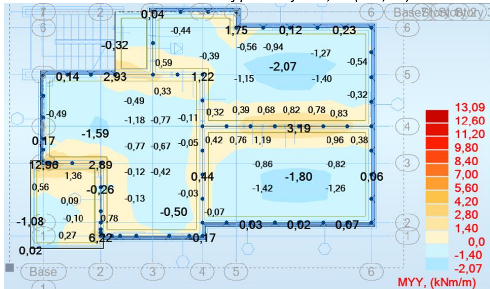
Slika 6.6 Armatura u međukatnoj ploči smjer A_{s,y-y} ( \text{cm}^2/\text{m} ) za GSN-1
