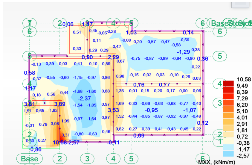
Slika 6.5 Armatura u krovnoj ploči smjer A_{s,x-x} ( cm^2/m ) za GSN-1
