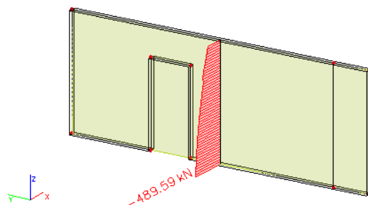
Slika 11.18 Maksimalna uzdužna sila za seizmičku kombinaciju KSY
