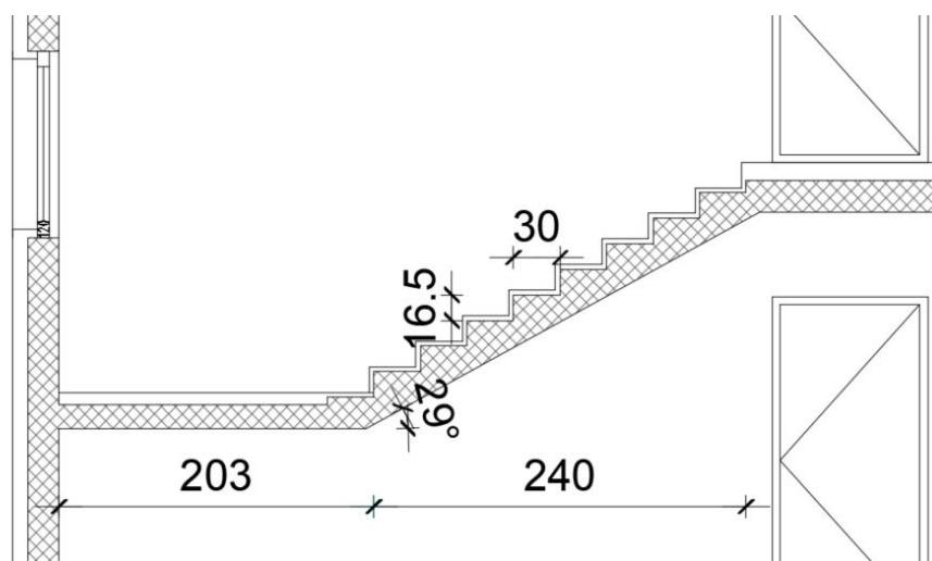
Slika 12.1 Detalj stubišta
