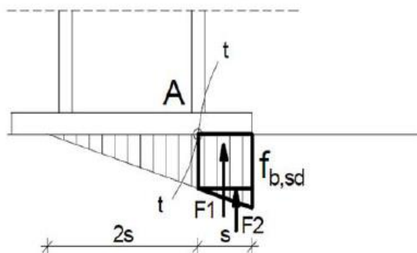
Slika 6.2 Pritisak po omotaču rupe
