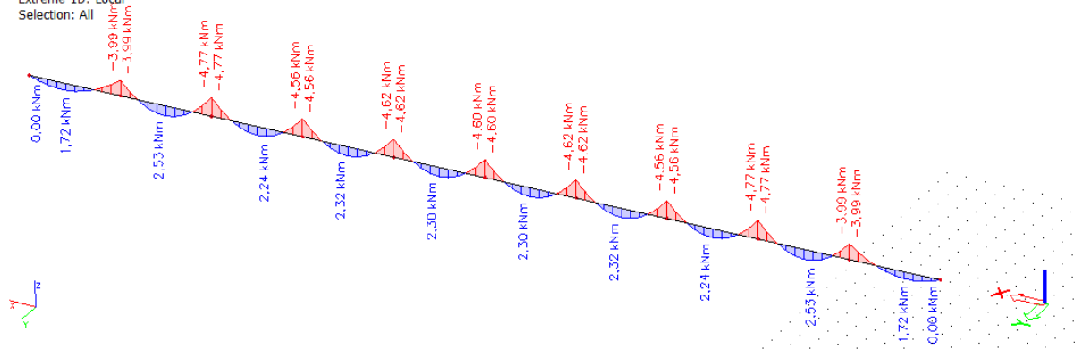
Slika 4.27 Momentni dijagram oko osi z uslijed stalnog opterećenja
