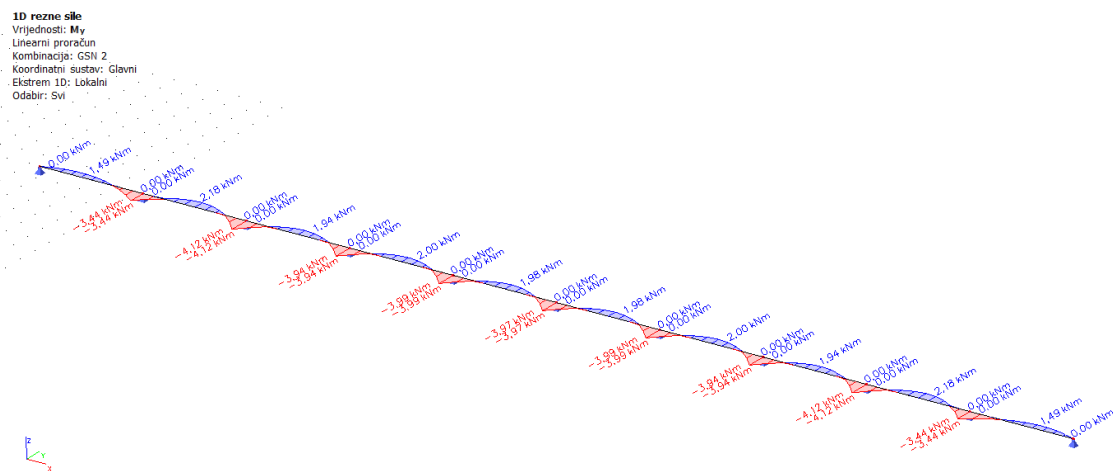
Slika 4.38 Momentni dijagram oko osi y za 2. kombinaciju
