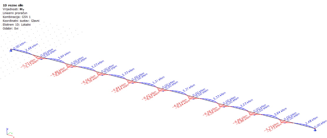
Slika 4.34 Momentni dijagram oko osi y za 1. kombinaciju
