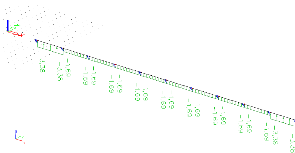
Slika 4.13 Djelovanje odizuceg vjetra na krovnu podroznicu
