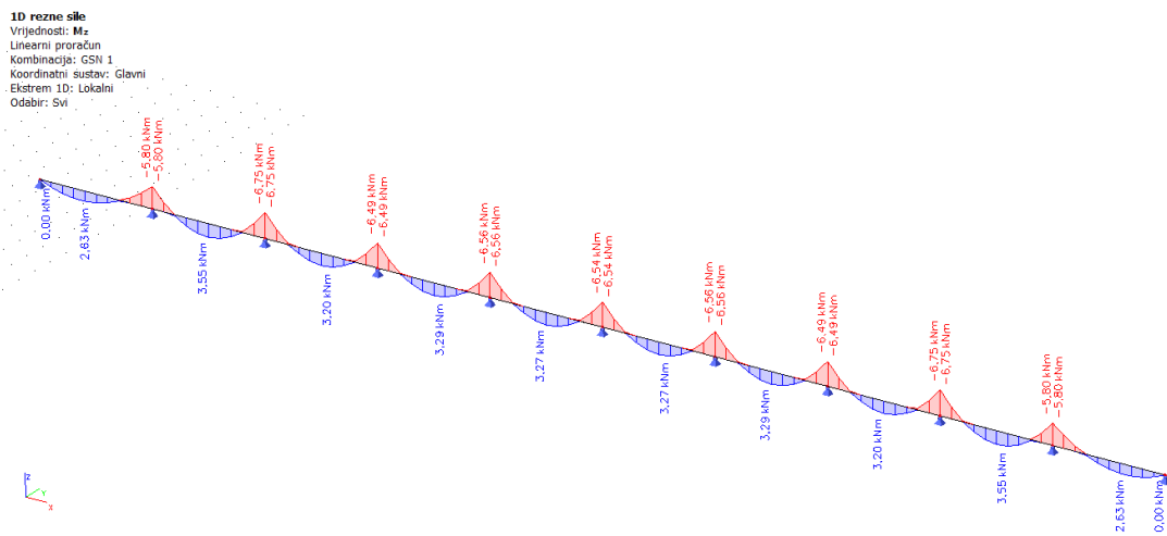
Slika 4.32 Momentni dijagram oko osi z za 1. kombinaciju
