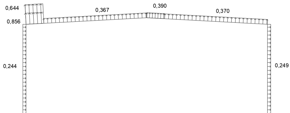
Slika 2.13 Rezultati pritiska vjetra za 3. kombinaciju
