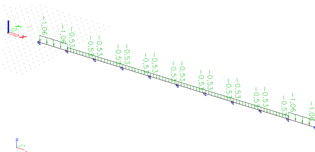
Slika 4.12 Djelovanje pritisakajuceg vjetra na krovnu podroznicu
