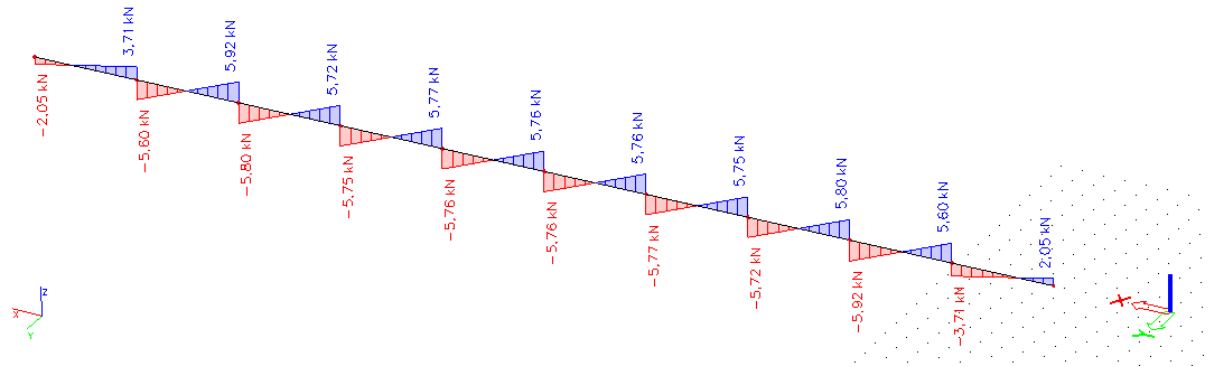
Slika 4.28 Dijagram poprečnih sila oko osi y uslijed djelovanja stalnog opterećenja
