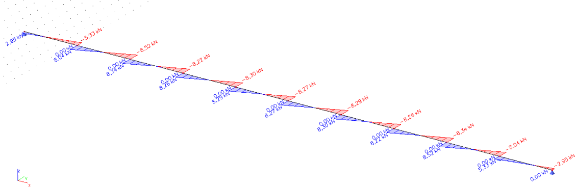
Slika 4.35 Dijagram poprečnih sila u smjeru osi z za 1. kombinaciju
