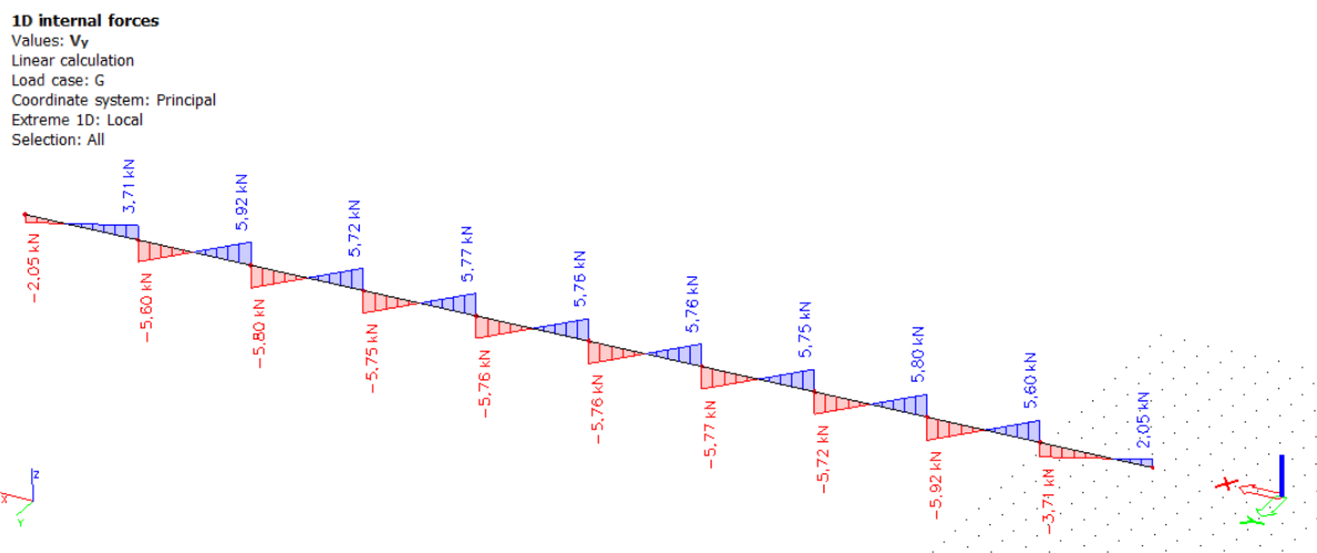
Slika 4.28 Dijagram poprečnih sila oko osi y uslijed djelovanja stalnog opterećenja
