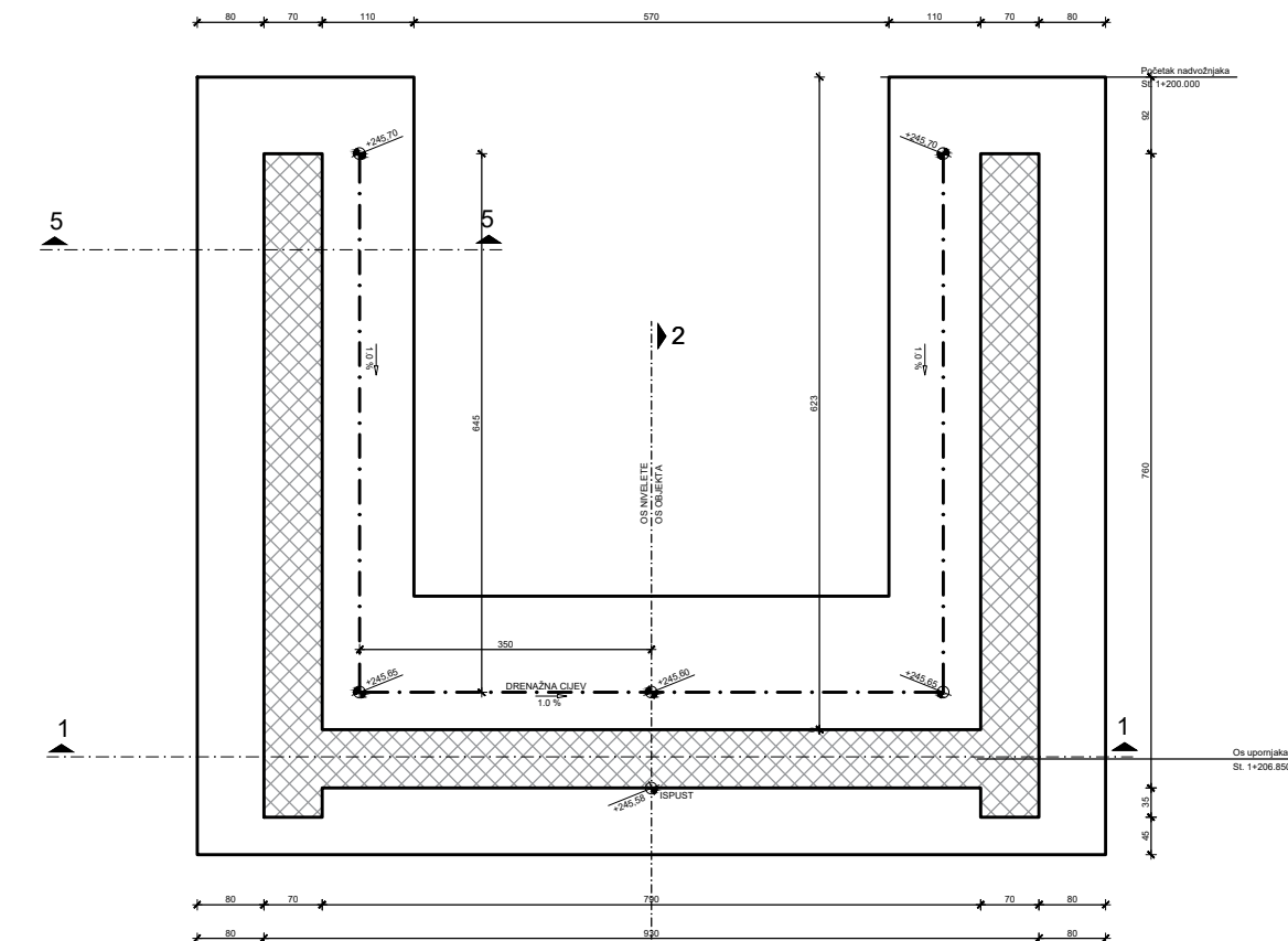
Presjek 3-3
