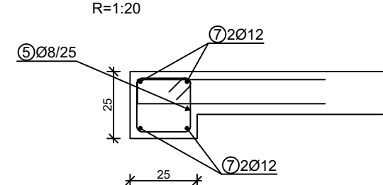
DETALJ HORIZONTALNIH SERKLAŽA M 1:20 (D-D)
