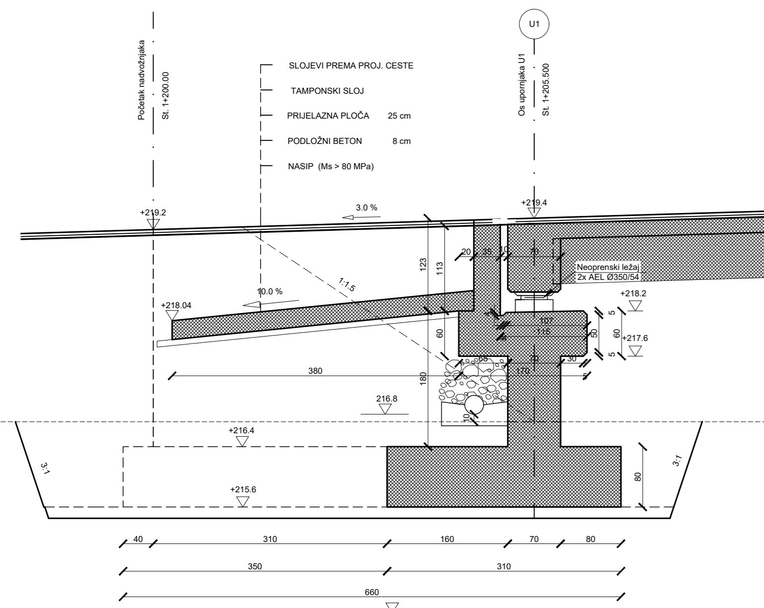
Presjek 3-3
