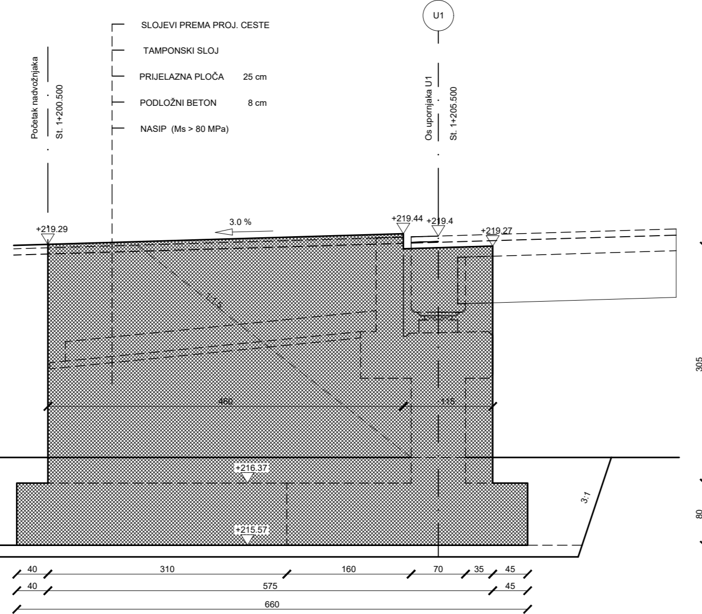
Presjek 5-5
