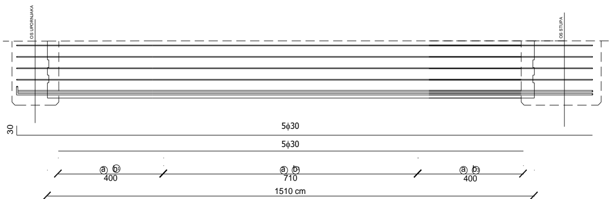
Slika 31. Prikaz armiranja uzdužnog nosača u polju
