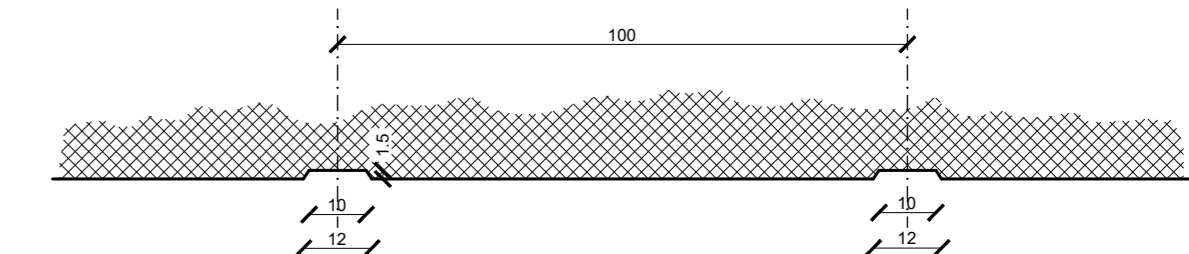
Detalj kanelura
