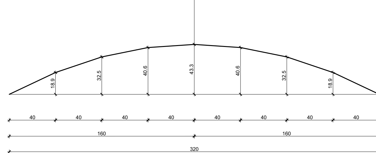
SHEMA NADVIŠENJA OPLATE NOSAČA
