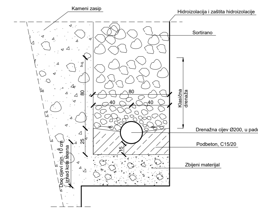
Detalj drenaže
