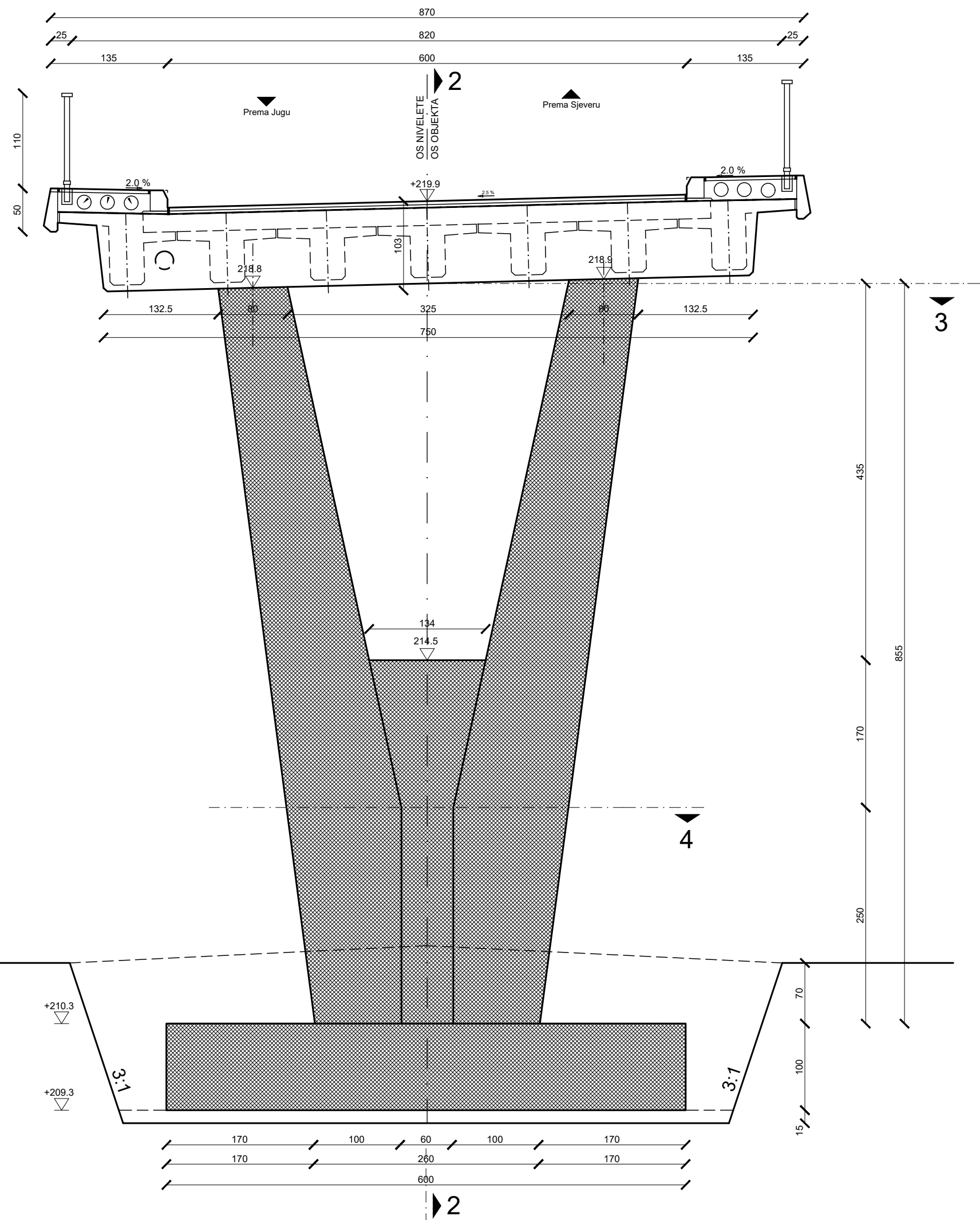
Presjek 1-1
