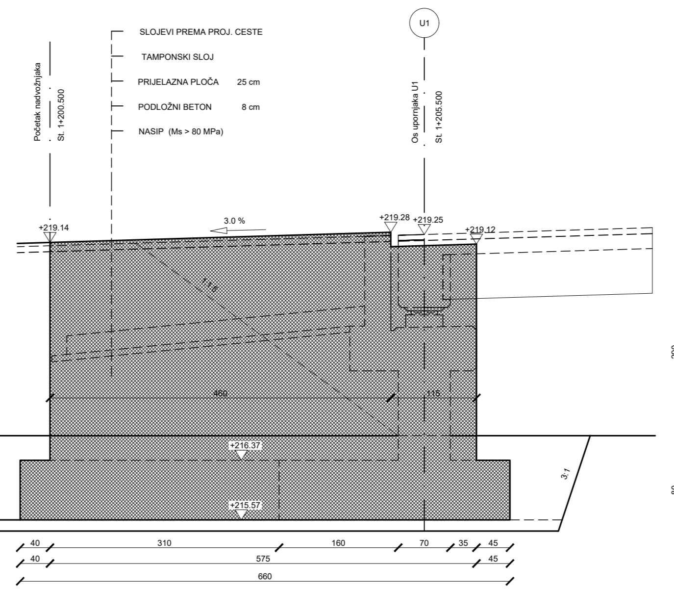
Presjek 6-6
