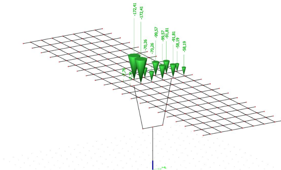
Slika 26. Prikaz opterećenja tipskog vozila za maksimalnu poprečnu silu pri stupu
