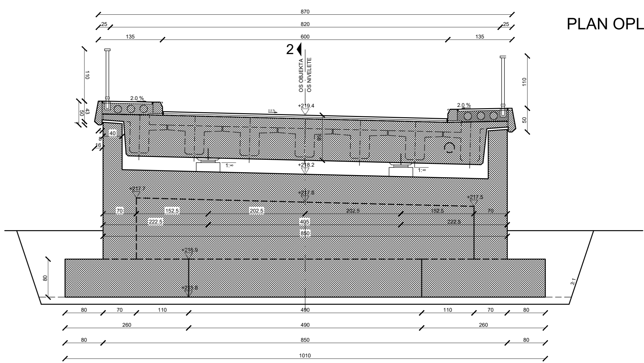
Presjek 1-1
