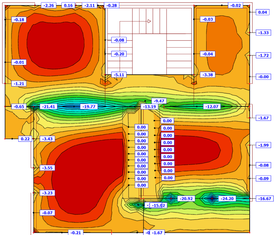
Moment m_y
