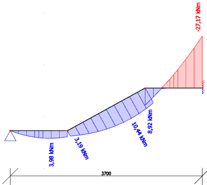
Slučaj kad je gornji podest upet u zid
