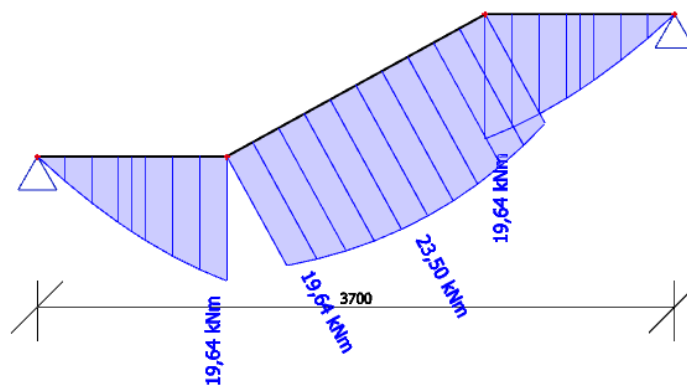
Slučaj kad je stubište slobodno oslonjeno
