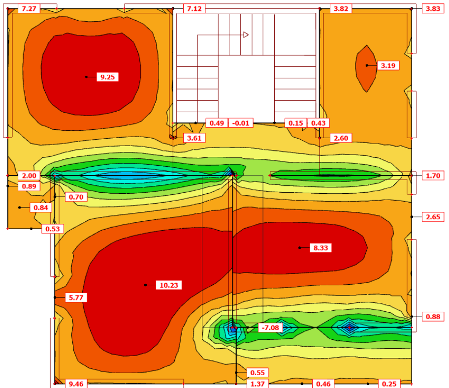
Moment m_y
