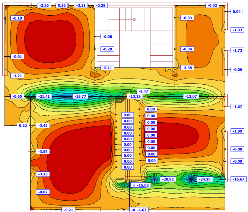
Moment m_y
