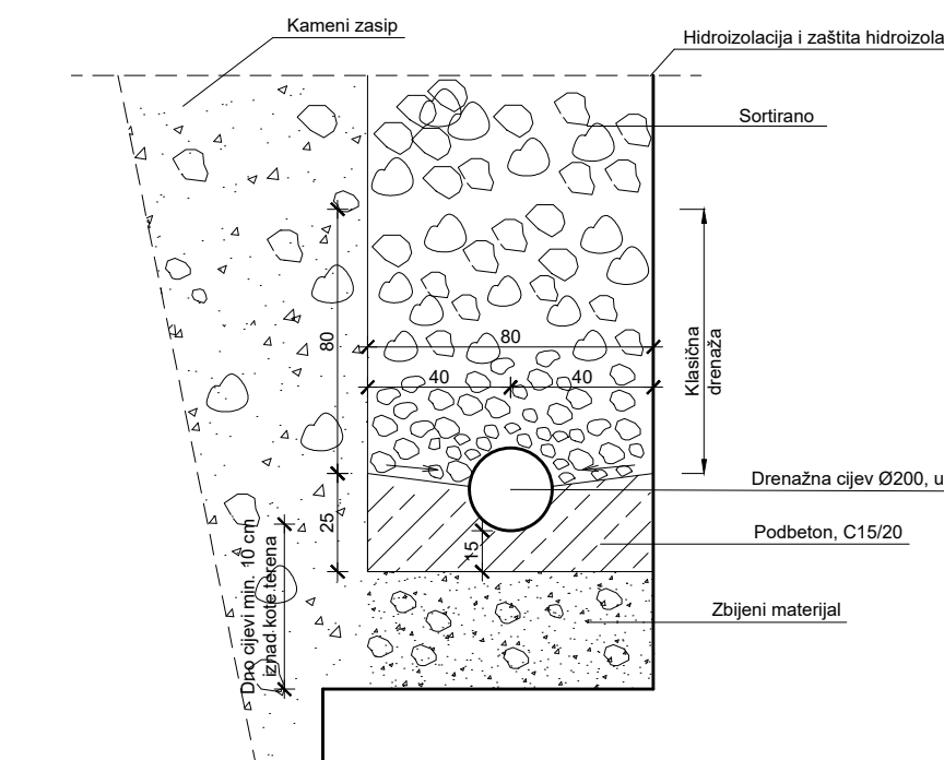
DETALJ DRENAŽE
