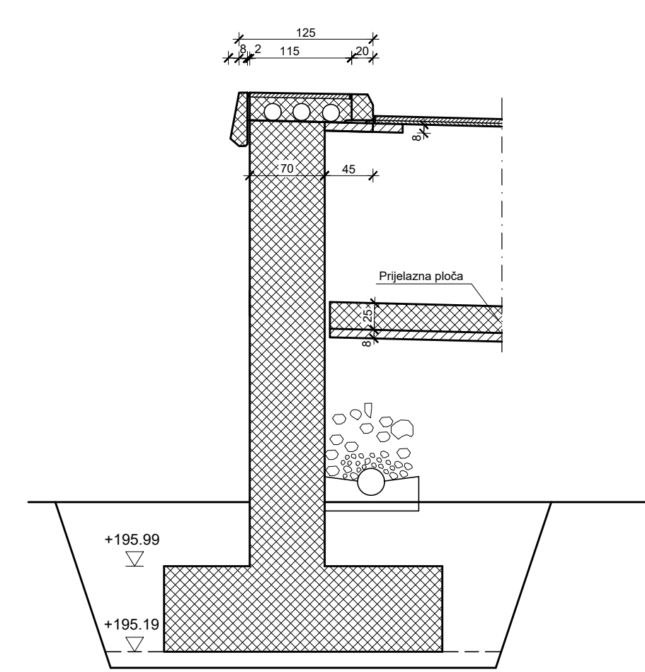
Presjek 7-7
