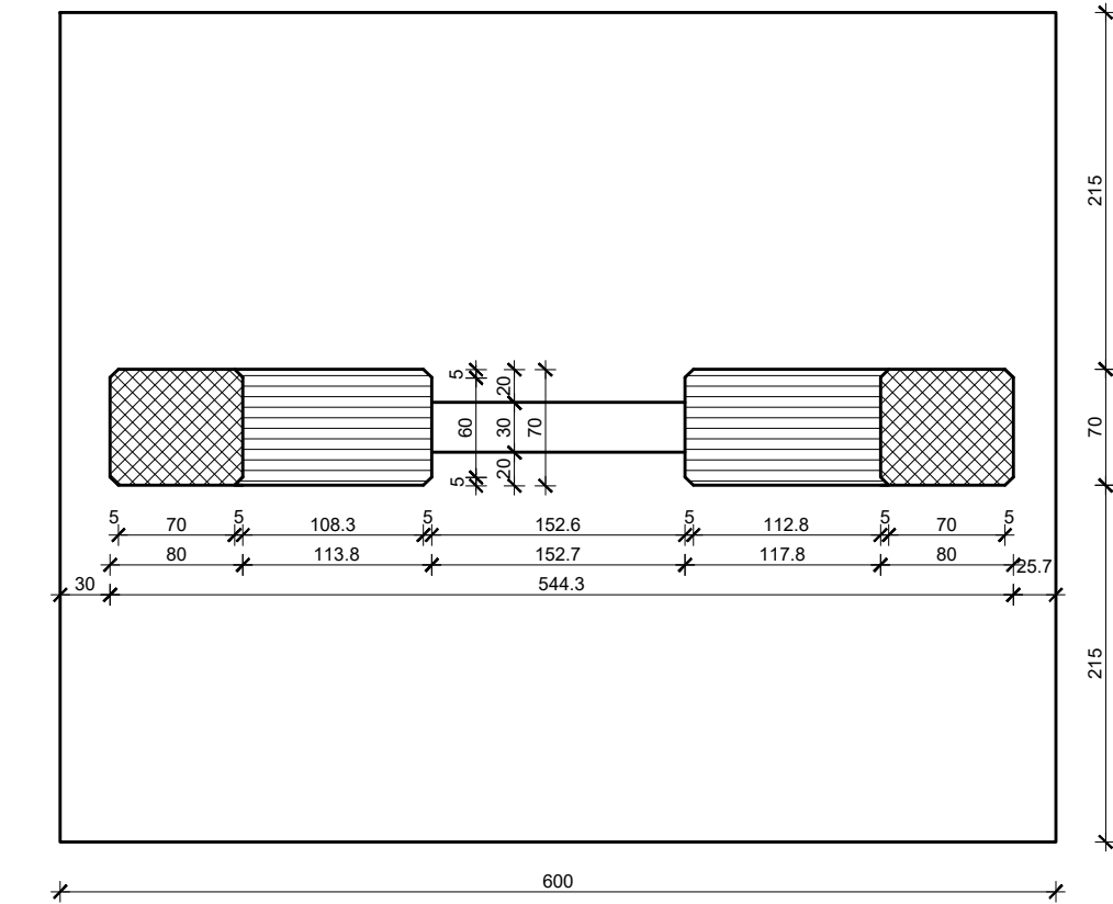
Presjek 4-4
