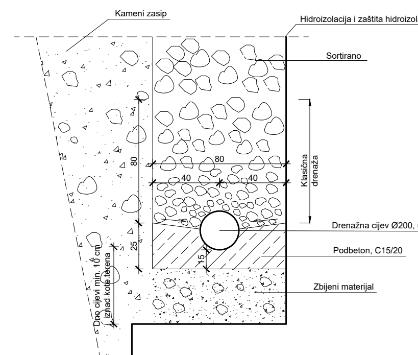
Detalj drenáže
