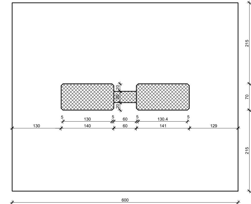
Presjek 4-4
