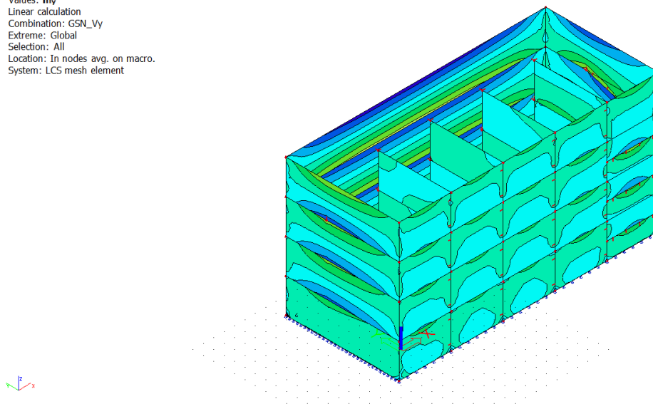
Slika 11.16: Moment M_y (kNm) – GSN Vy
