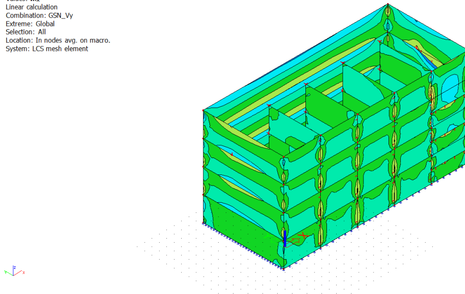
Slika 11.15: Moment M_x (kNm) – GSN Vy
