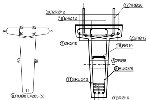
PRESJEK 1-1
