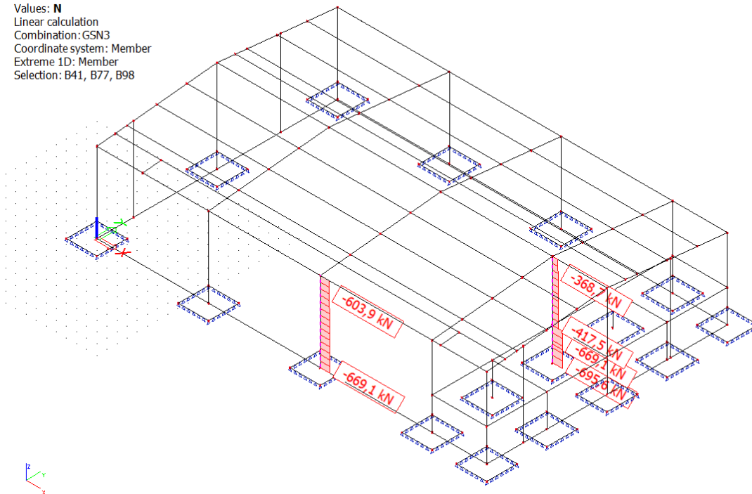
Slika 9.11 Prikaz uzdužne sile za odabrane stupove S10 i S2 za GSN3
