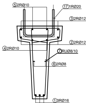
PRESJEK 2-2
