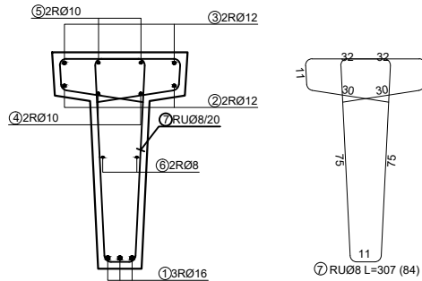
PRESJEK 3-3
