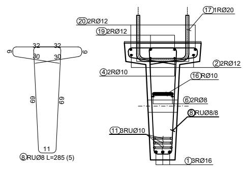
PRESJEK 1-1
