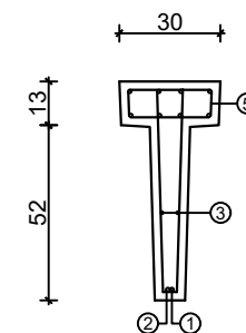
PRESJEK A-A
