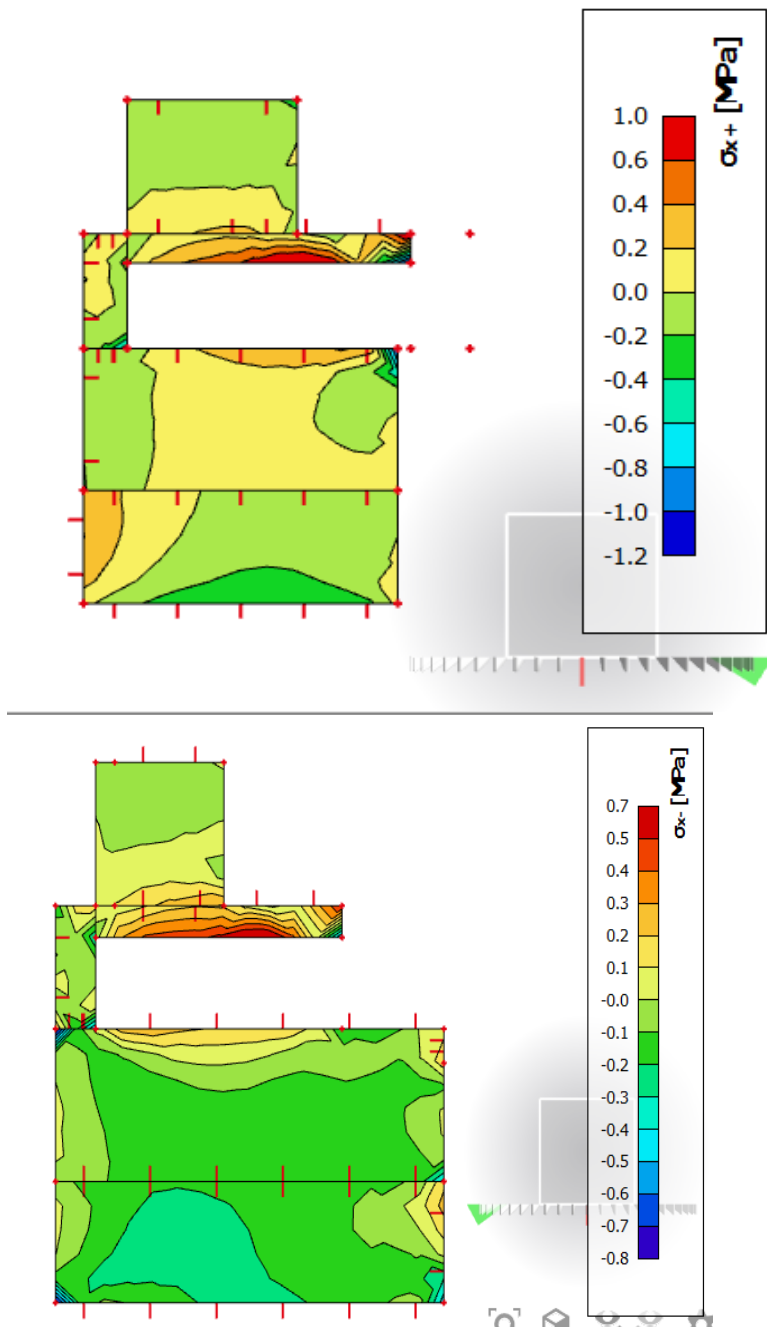
Slika 8.16. Naprezanja u smjeru x
