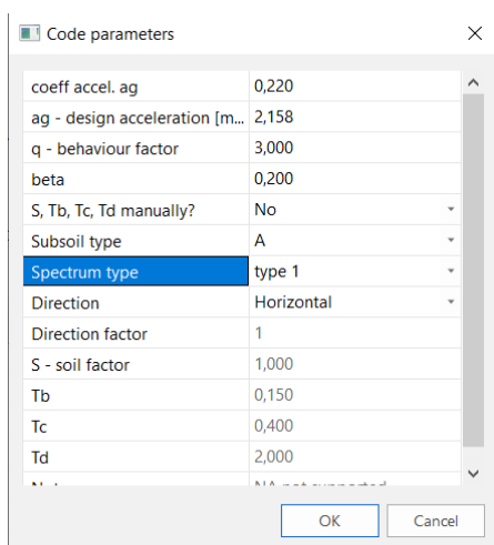
Slika 4.12 Ulazni parametri za proračun
