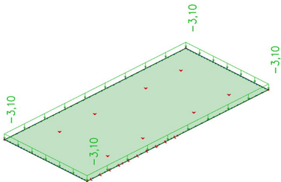
Slika 6.42. Dodatno stalno opterećenje ( \text{kN/m}^2 )
