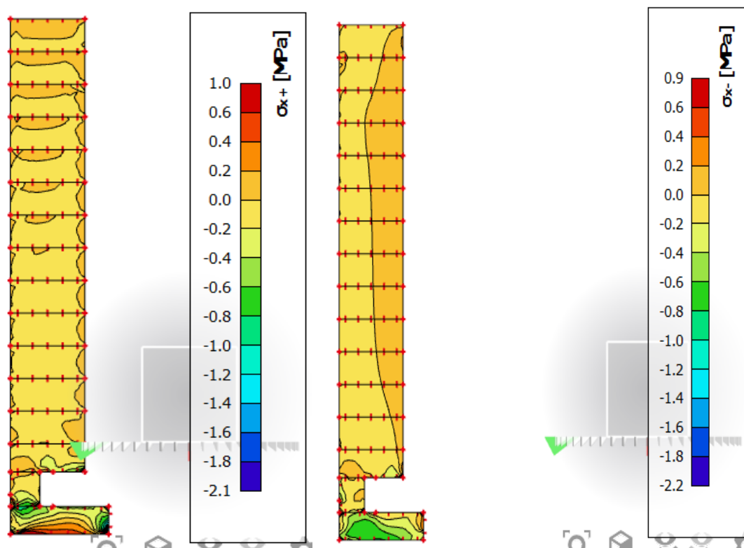
Slika 8.33. Napreznja u smjeru x
