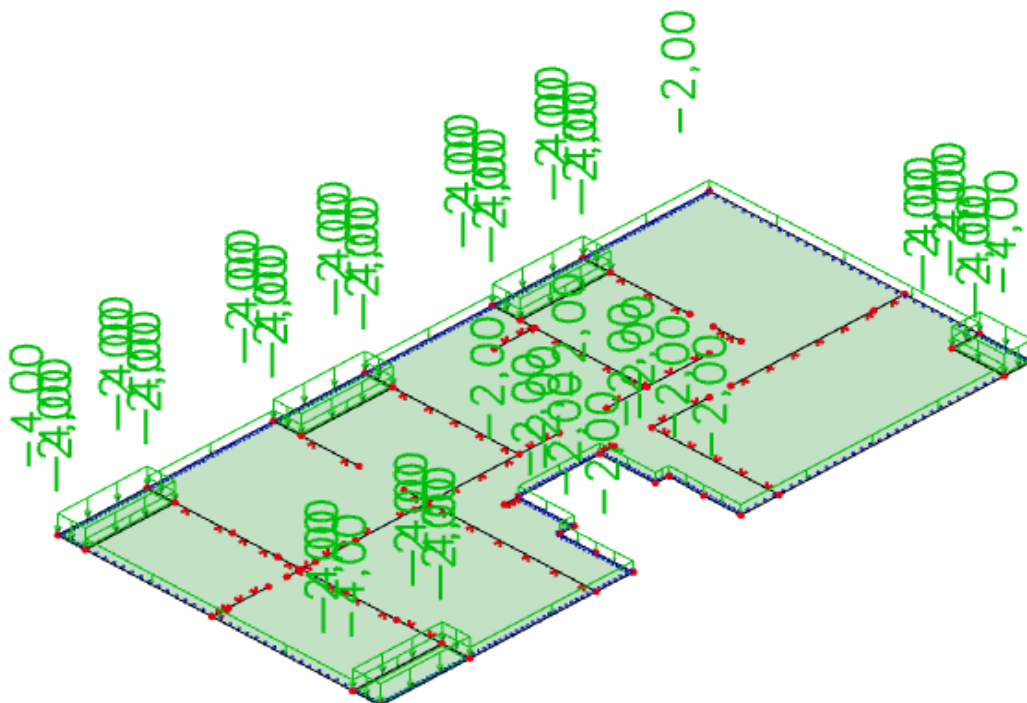
Slika 6.28. Dodatno stalno opterećenje (kN/m 2 )
