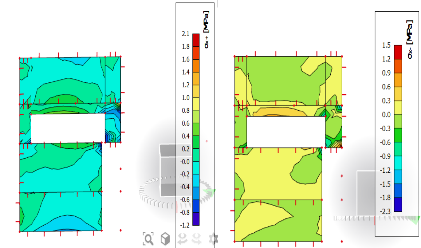
Slika 8.21. Napreznja u smjeru x
