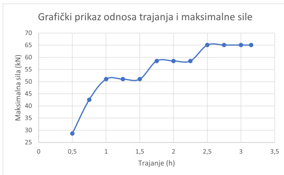
Slika 93 Grafički prikaz odnosa trajanja simulacije i maksimalne sile
